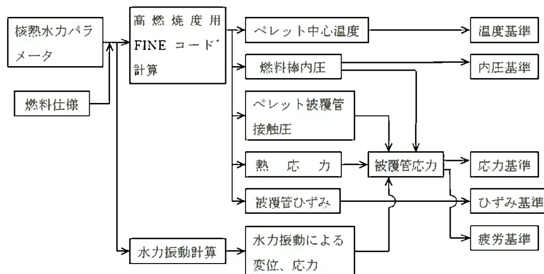
燃料棒強度評価フロー図
