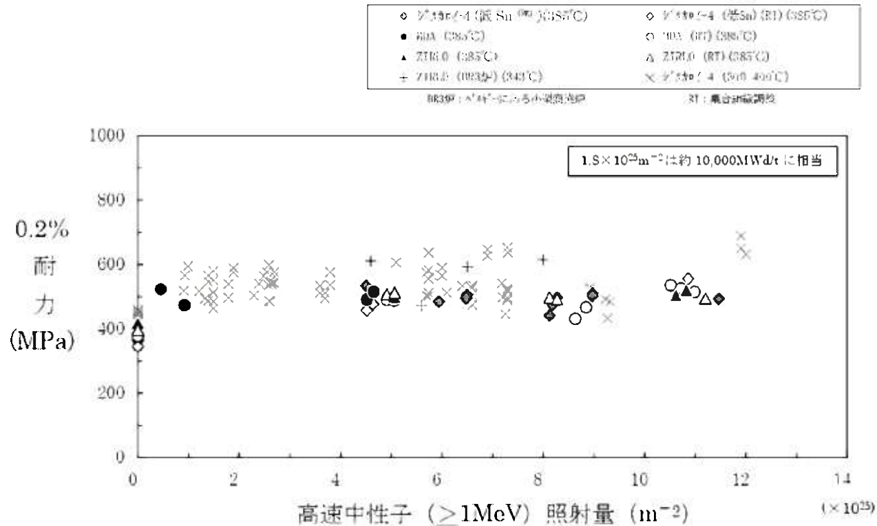
MDA及びZIRLO被覆管の機械特性
