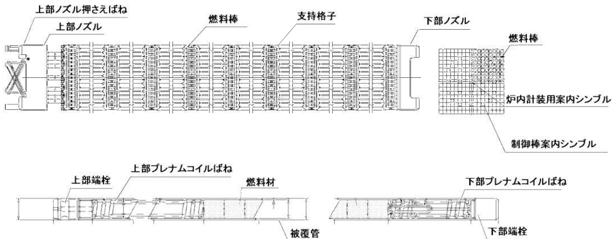
燃料体の構造概要図
