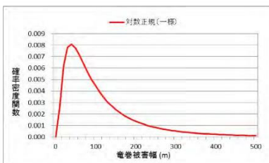
第2.2.2.2-5図 被害幅の確率密度分布
