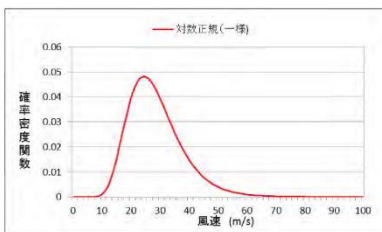
第2.2.2.2-3図 竜巻風速の確率密度分布
