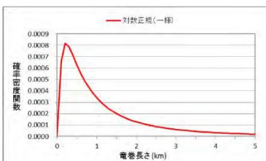
第2.2.2.2-7図 被害長さの確率密度分布
