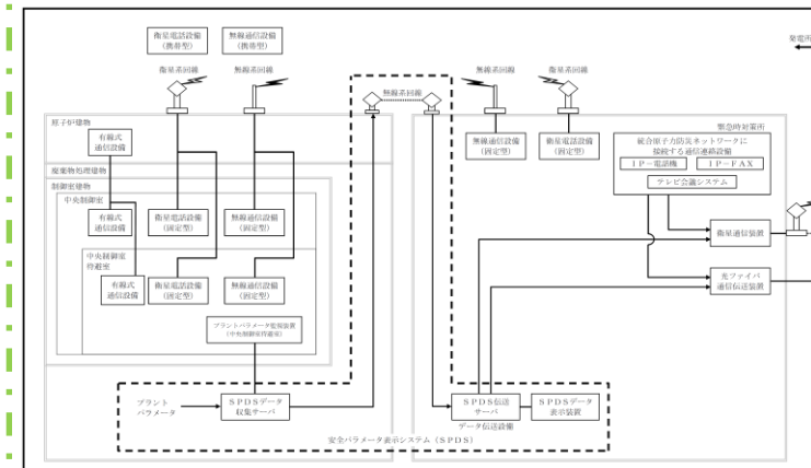
図 2.4-20 プラントパラメータ監視装置 (中央制御室待避室) のデータ伝送 概要図
