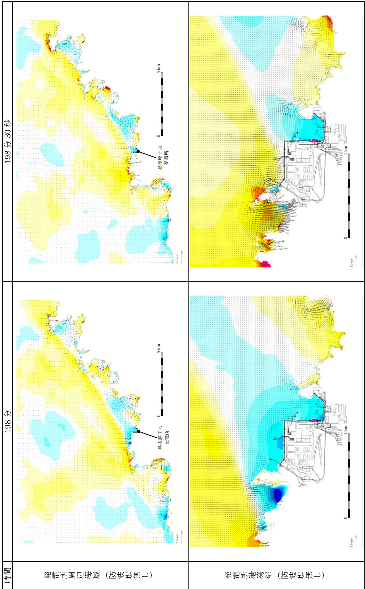
第 5 図 (29) 基準津波 5 の水位変動・流向ベクトル
