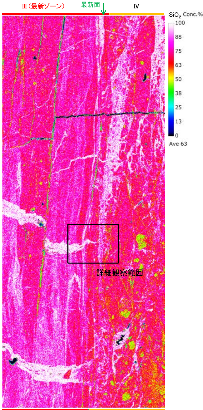
SiO 2
