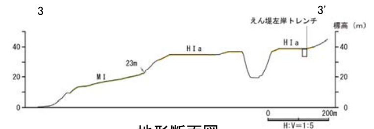
地形断面図
