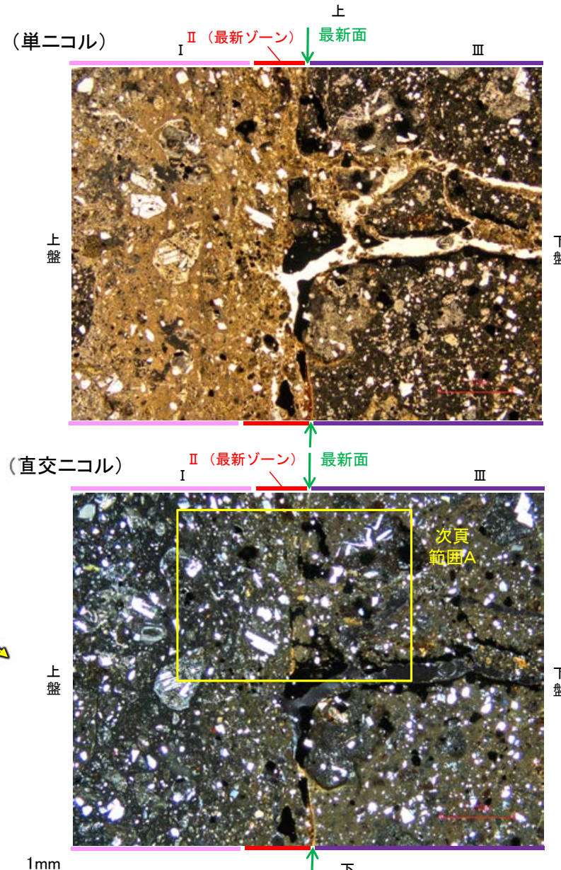
観察用薄片写真(H- -0.3-80_107R) (拡大)
