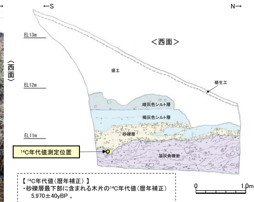
スケッチ(事務本館前トレンチ 西面)
