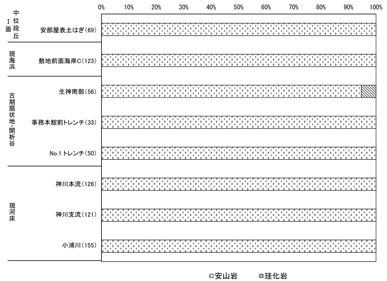
礫種検討結果 (地点名の横の括弧内に記載された数字は試料数)
