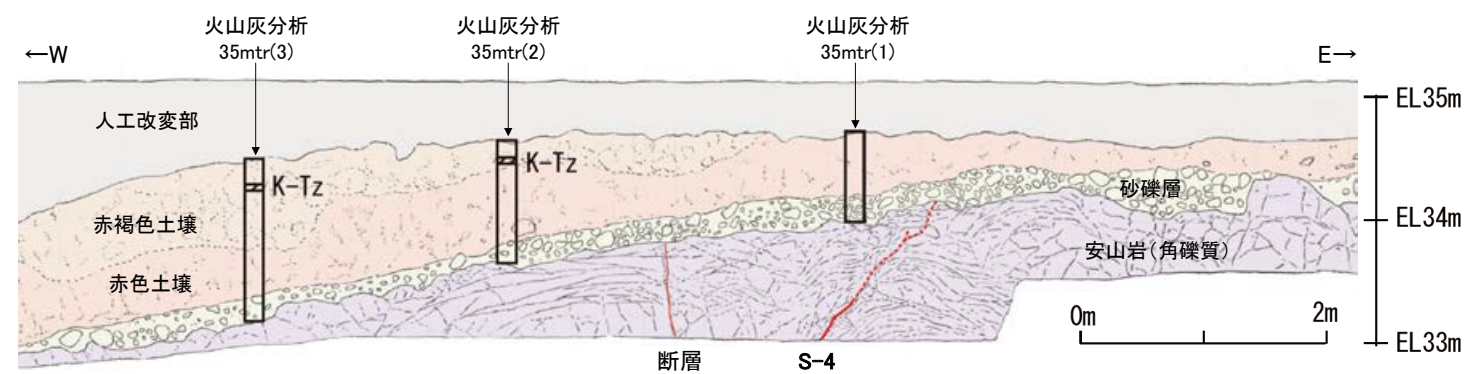
断層 S-4 スケッチ (35m盤トレンチ(B) 北面)
