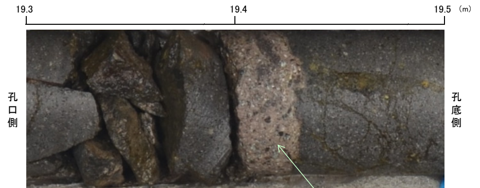
コア写真
