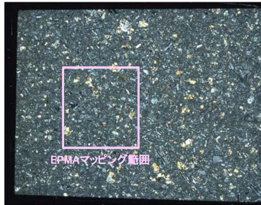
薄片写真
