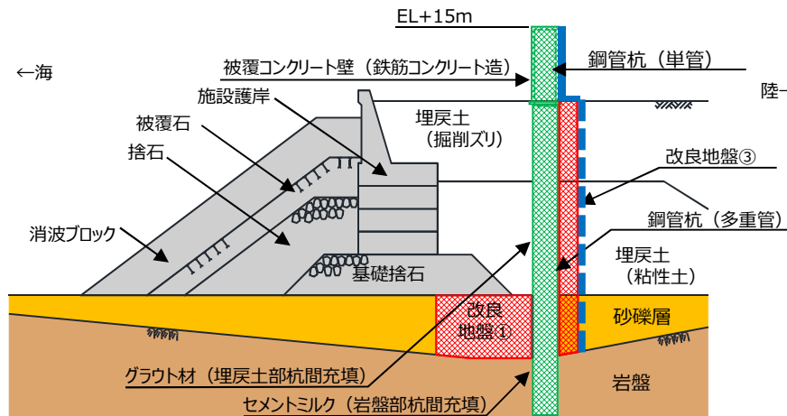
防波壁(多重鋼管杭式擁壁)(改良地盤部)における構造上のバウンダリ
