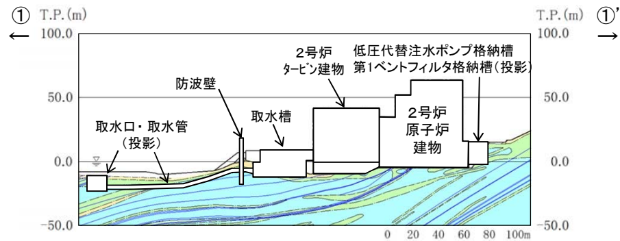
①-①' 断面図
