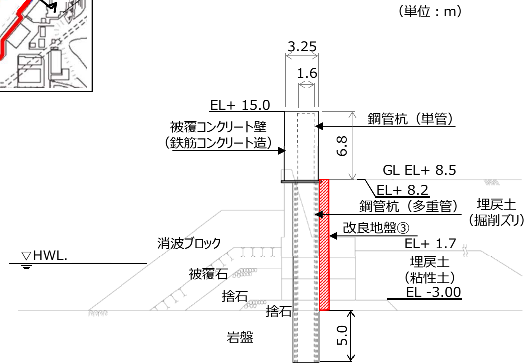
防波壁(多重鋼管杭式擁壁) 北東端部(⑤-⑤断面) 断面図
