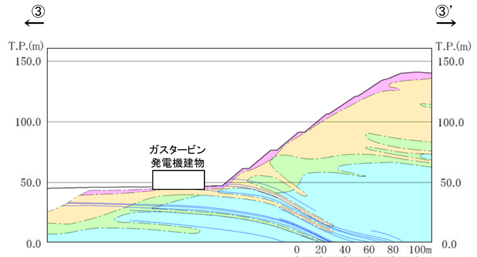
③-③' 断面図
