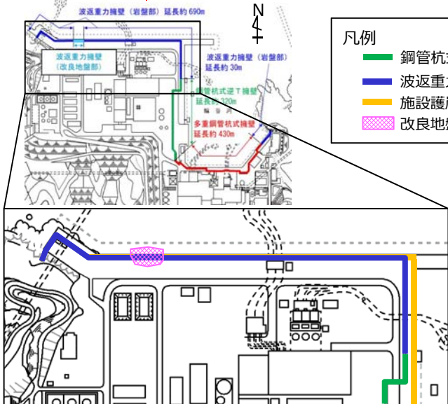
防波壁平面図(波返重力擁壁)
