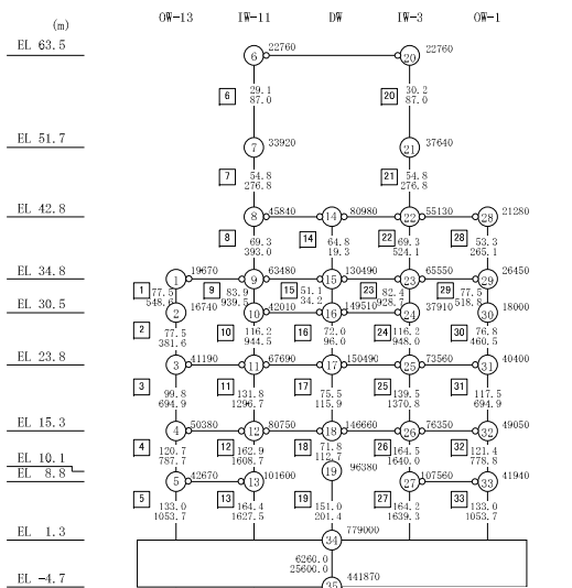
水平モデル(NS方向)
