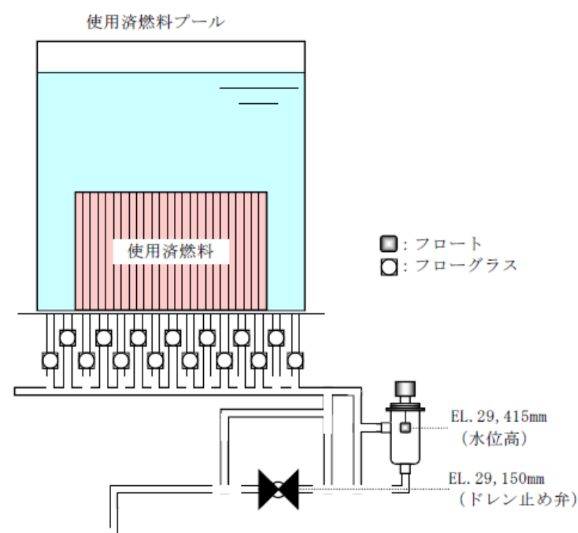
第1.2-5 図 使用済燃料プールライナードレン漏えい検知の警報設定値
