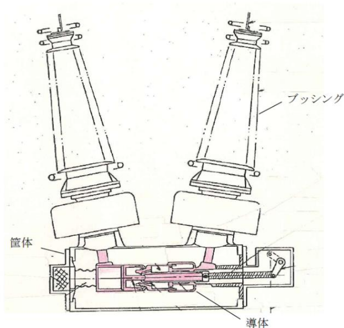
第2-6 図 GCB 構造概要
