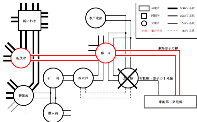
第2.2.2-4図 茨城変電所全停時の電力供給系統
