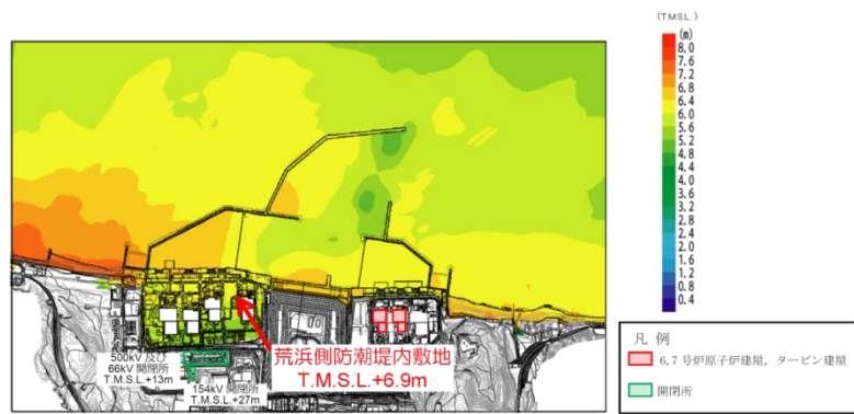
第 2.2.4-41 図 柏崎刈羽原子力発電所の敷地高さと各施設との関係
