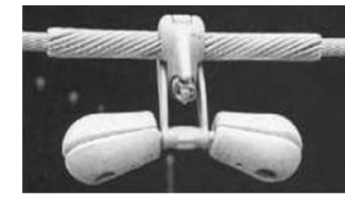
ねじれ防止ダンパー
