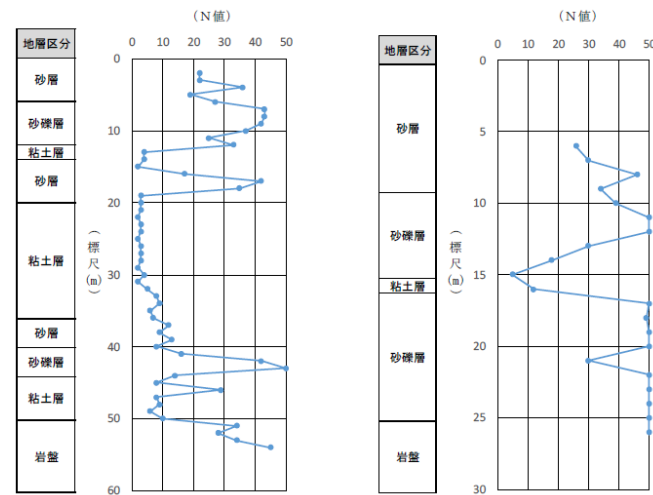
275kV 超高压開閉所付近 154kV 特別高压開閉所付近
