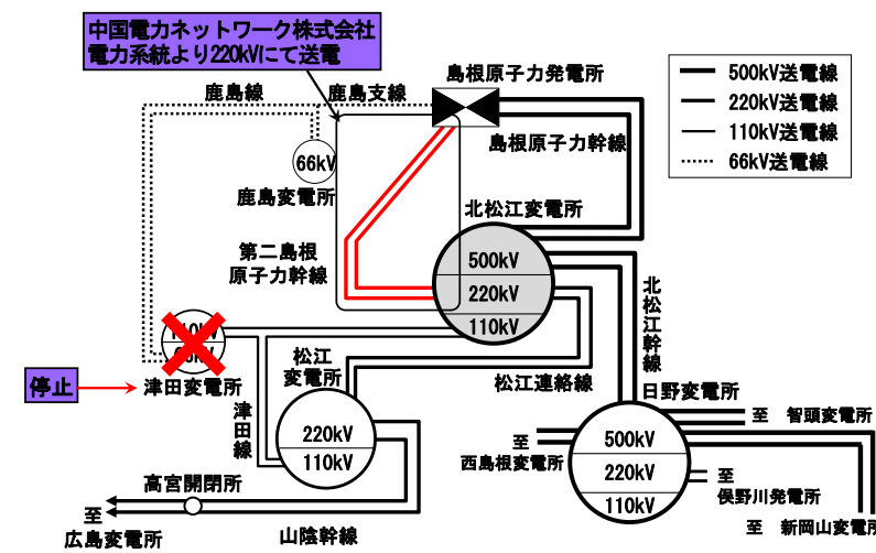
第2.2.2-7図 津田変電所全停時の供給系統
