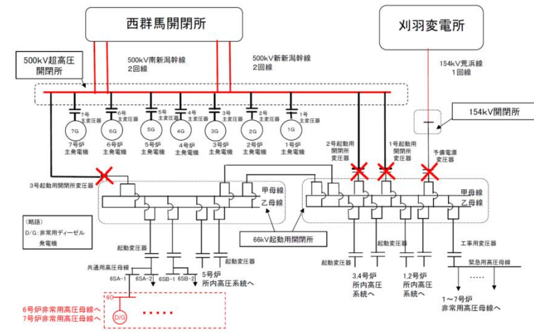
第2.2.4-5図 起動用開閉所変圧器及び予備電源変圧器故障時の電力供給
