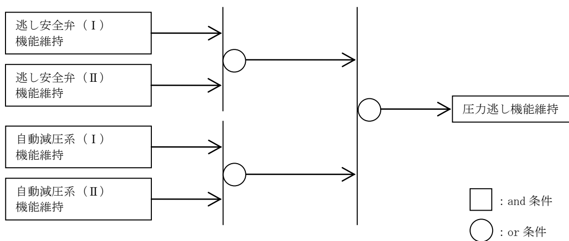
図 4 安全機能判定フロー (圧力逃し機能)
