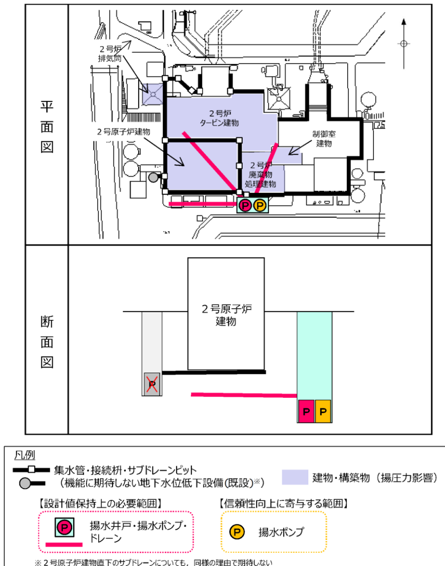
図10-6 地下水位低下設備の構成例
