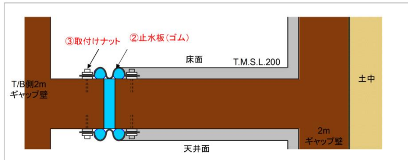
壁面断面図
