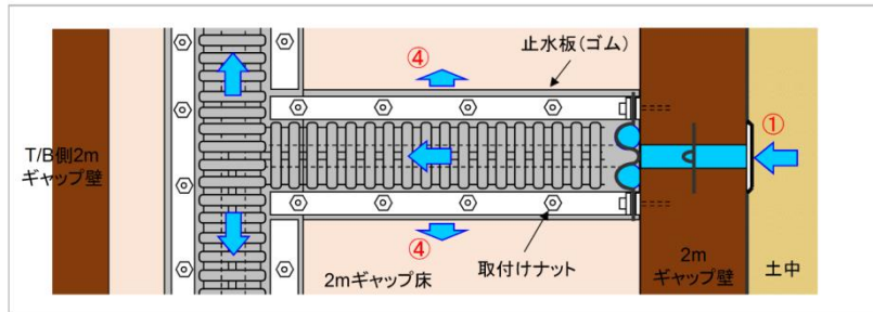
壁面断面図
