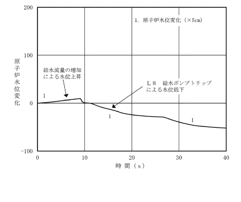
第 3 図 給水制御系の故障解析結果 (原子炉建屋起因) (1/2)
