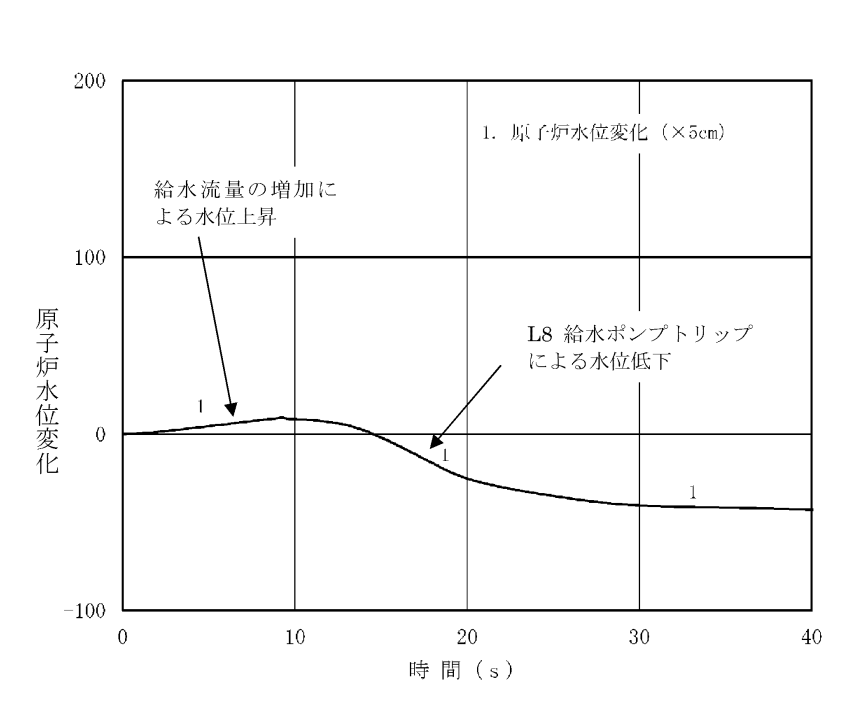
図 6-7 R/Bにおける内部溢水による事象変化 (原子炉水位) (給水制御系の故障)
