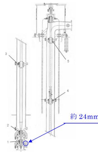
第6図 非常用ディーゼル発電機(高圧炉心スプレィ系ディーゼル発電機を含む。)用海水ポンプ断面図
