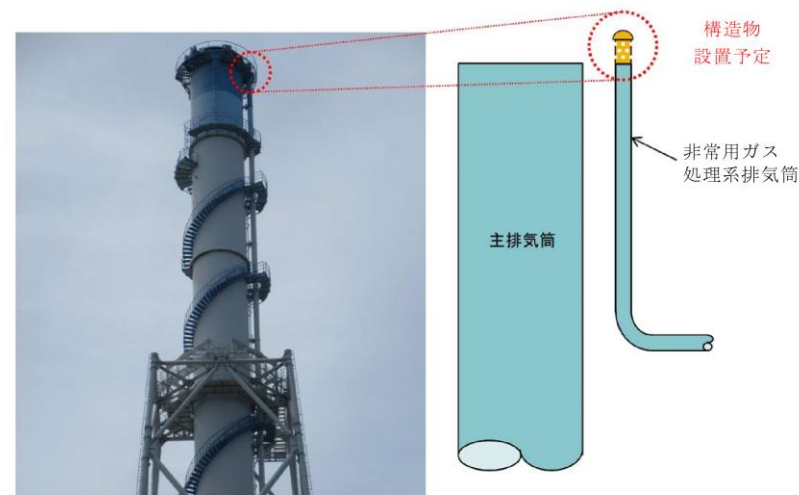
第 2 図 非常用ガス処理系排気筒 概略図
