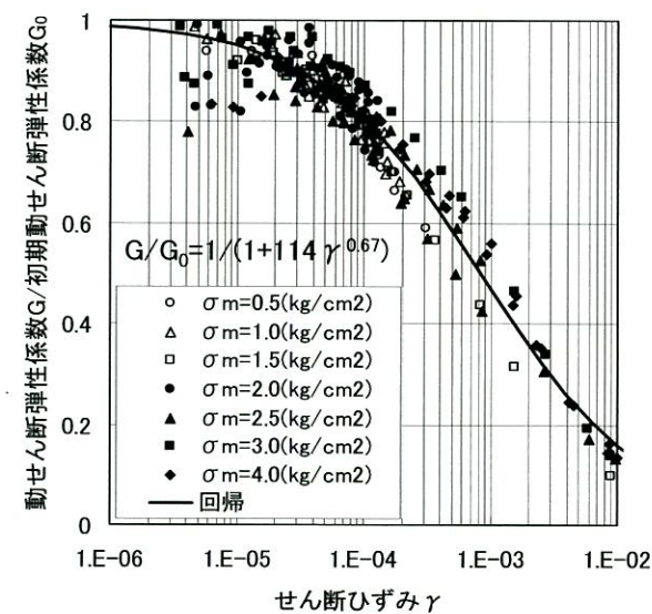
動的変形特性(G d /G 0 ~ gamma)
