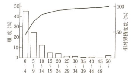
図-5.4 崩土の到達距離 (m) (1972～1982年) (16)
