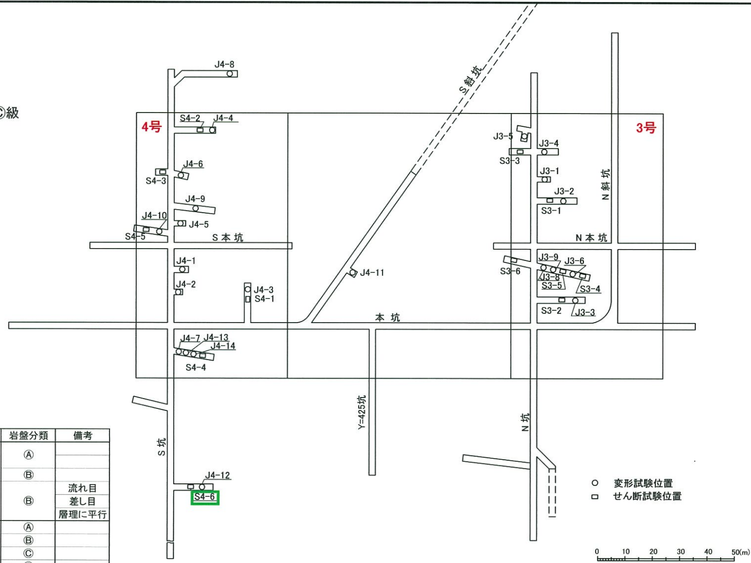
岩盤せん断試験実施位置(矽岩◎級)
