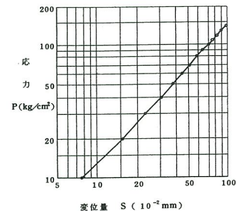
J4-9試験結果 (頁岩㊦級)
