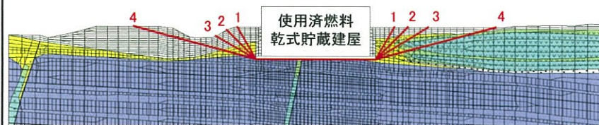
No.2) 建屋底面+断層・シームのすべり (Case1~4)
