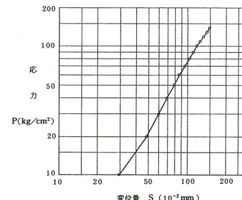
J3-6試験結果 (頁岩㊦級)
