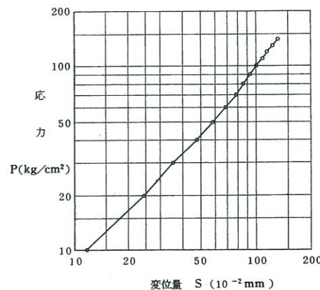
J3-4試験結果 (砂岩㊦級)
