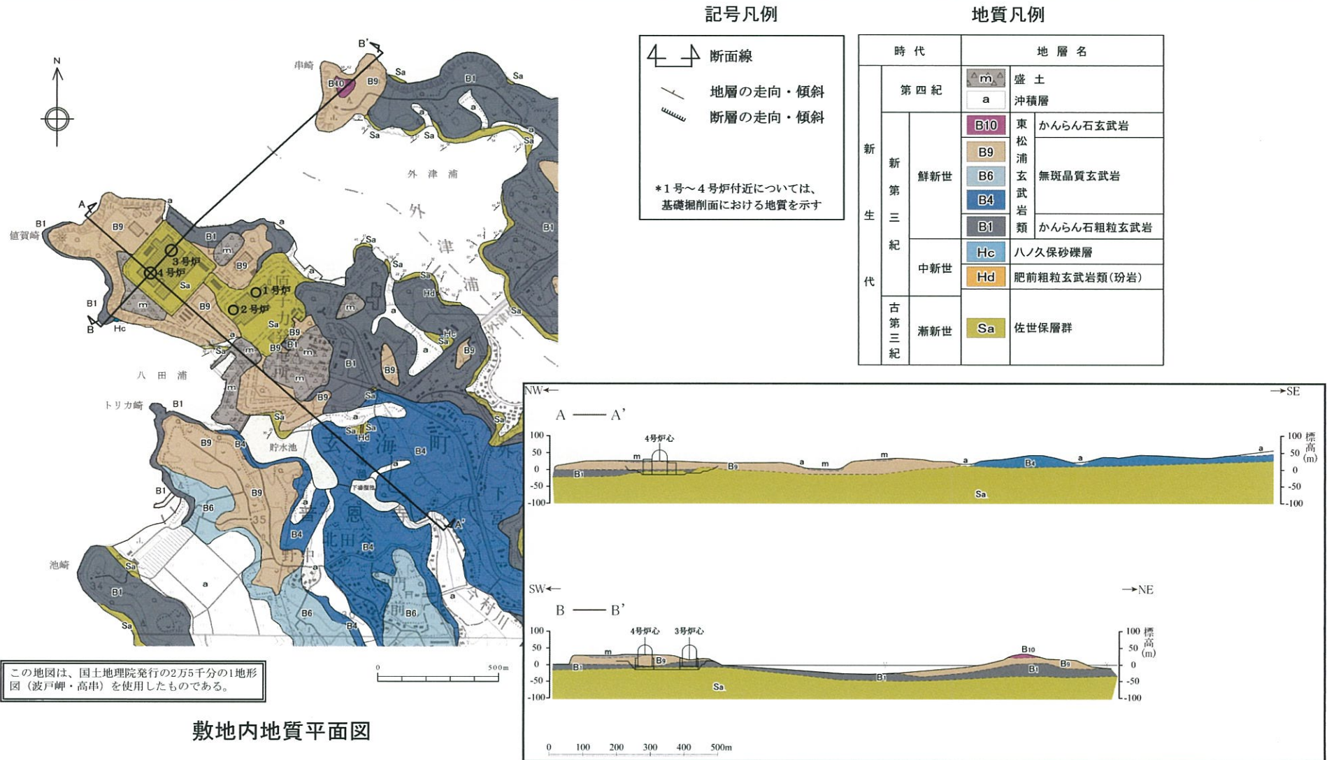
敷地内地質断面図
