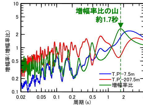
(1) S波増幅率
