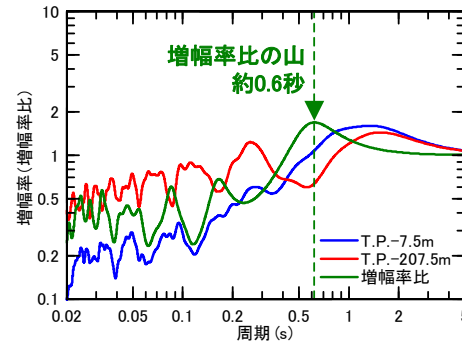
(2) P波増幅率
