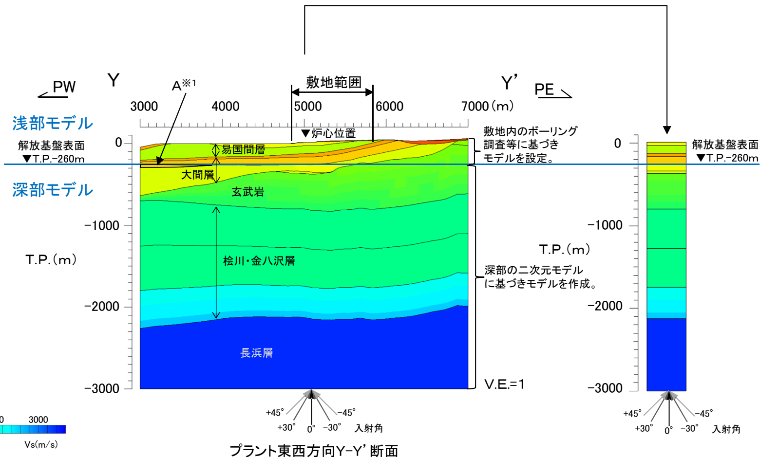
炉心位置の水平成層モデル※2
