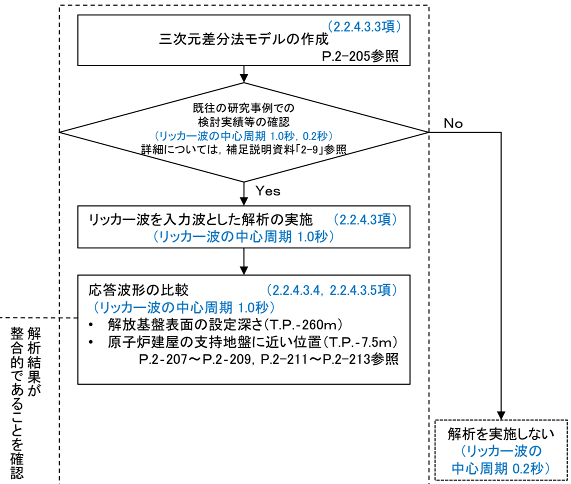
浅部の地下構造が地震動に及ぼす影響の検討フロー
