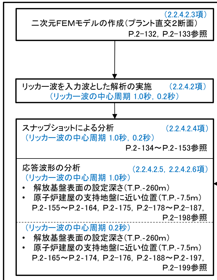
浅部の地下構造が地震動に及ぼす影響の検討フロー
