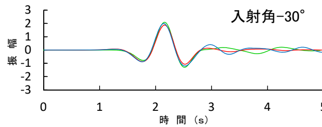
炉心位置の解放基盤表面での応答波形
