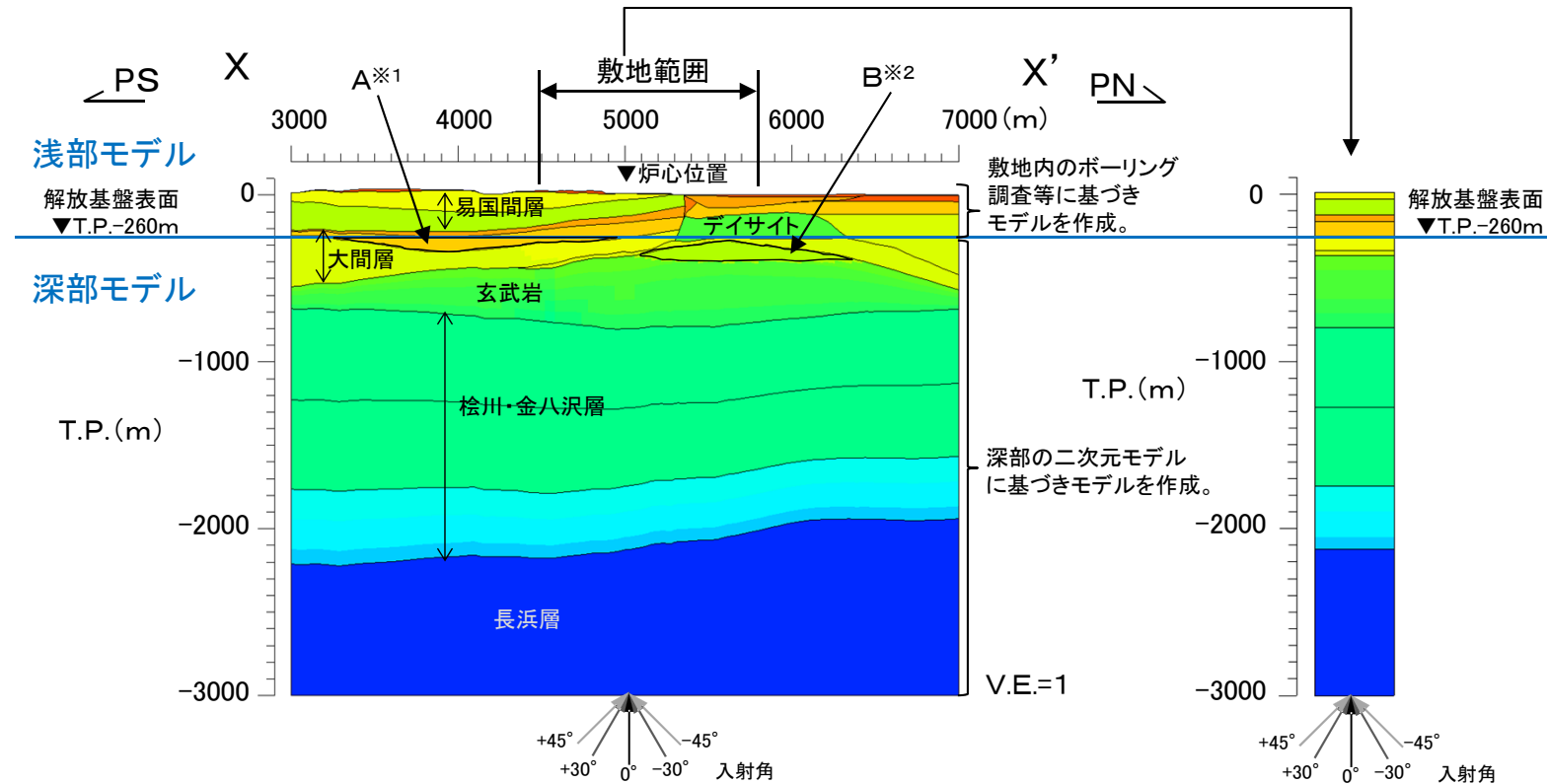
プラント南北方向X-X'断面 解放基盤表面以浅の構造を含む二次元FEMモデル
