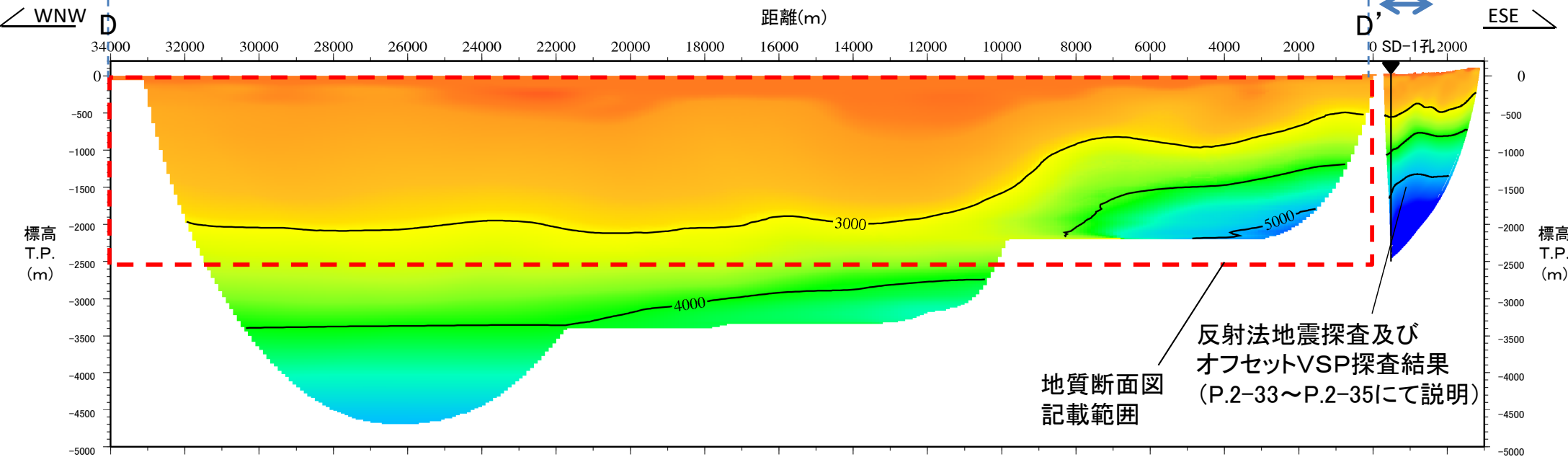
敷地周辺海域の屈折法地震探査及びオフセットVSP探査の速度構造図
