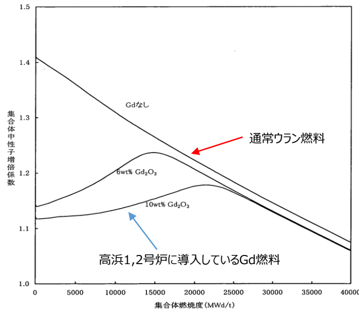
図※3:通常ウラン燃料とGd入り燃料の反応度 (中性子増倍率) (15×15型 20本Gd ウラン燃料棒 4.6wt% 235 U)
