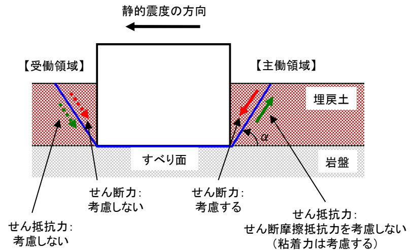
簡便法によるすべり安全率の算定方法 イメージ図
