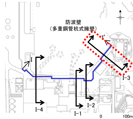
断面位置図
