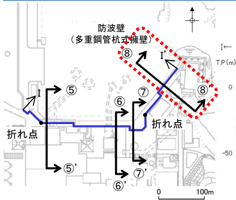
断面位置図
