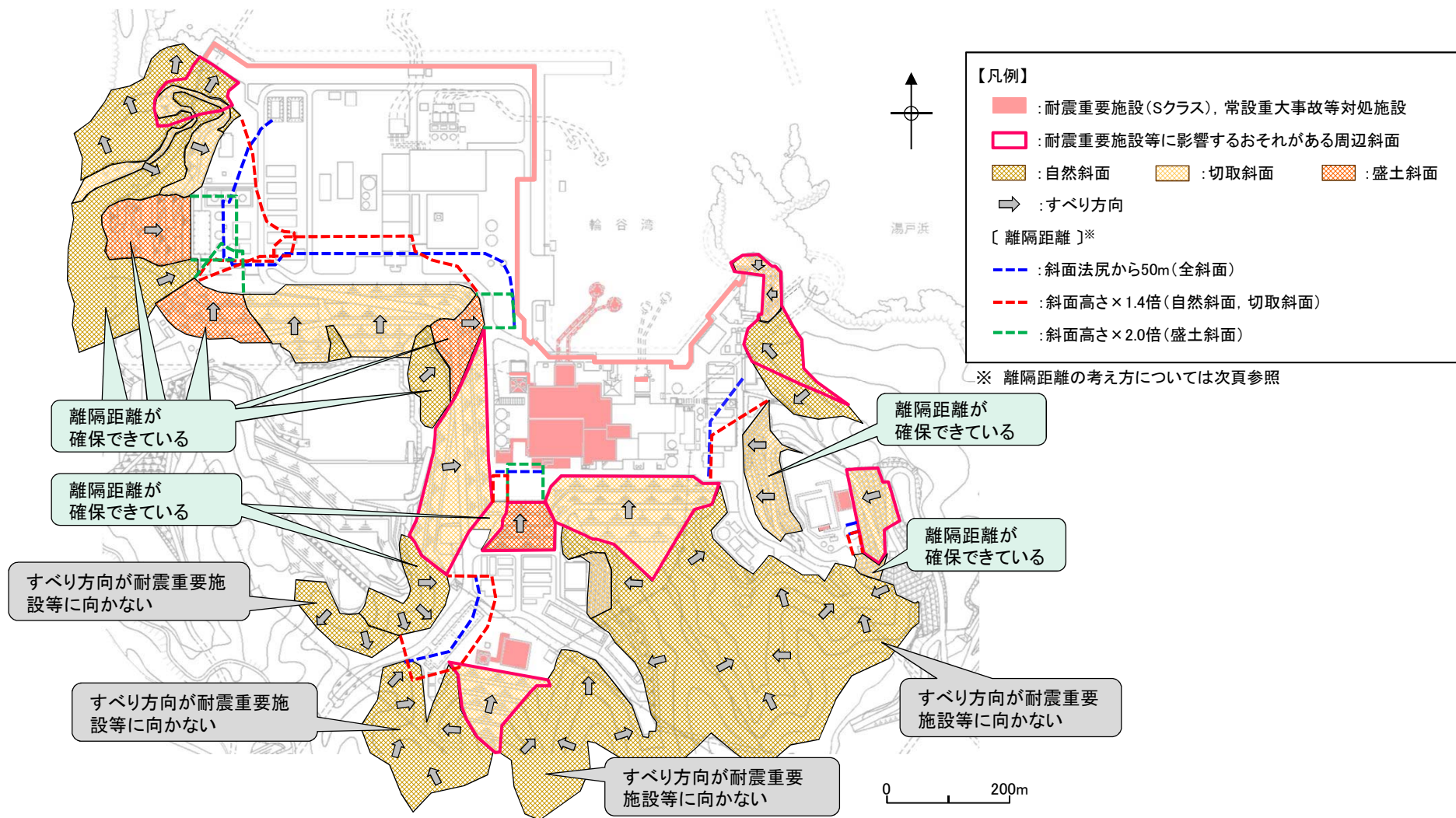
平面位置図
