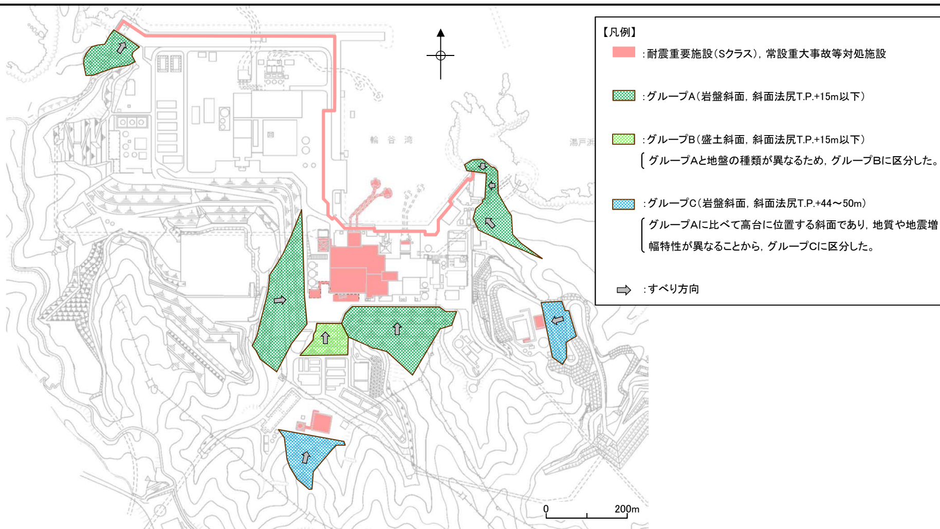
平面位置図
