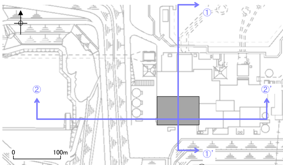
断面位置図
