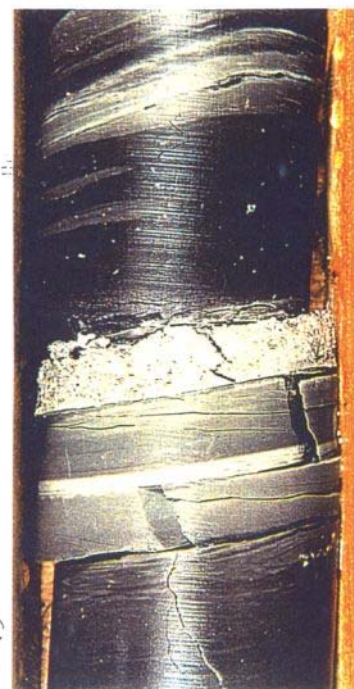
ボーリングコアにおけるシーム
