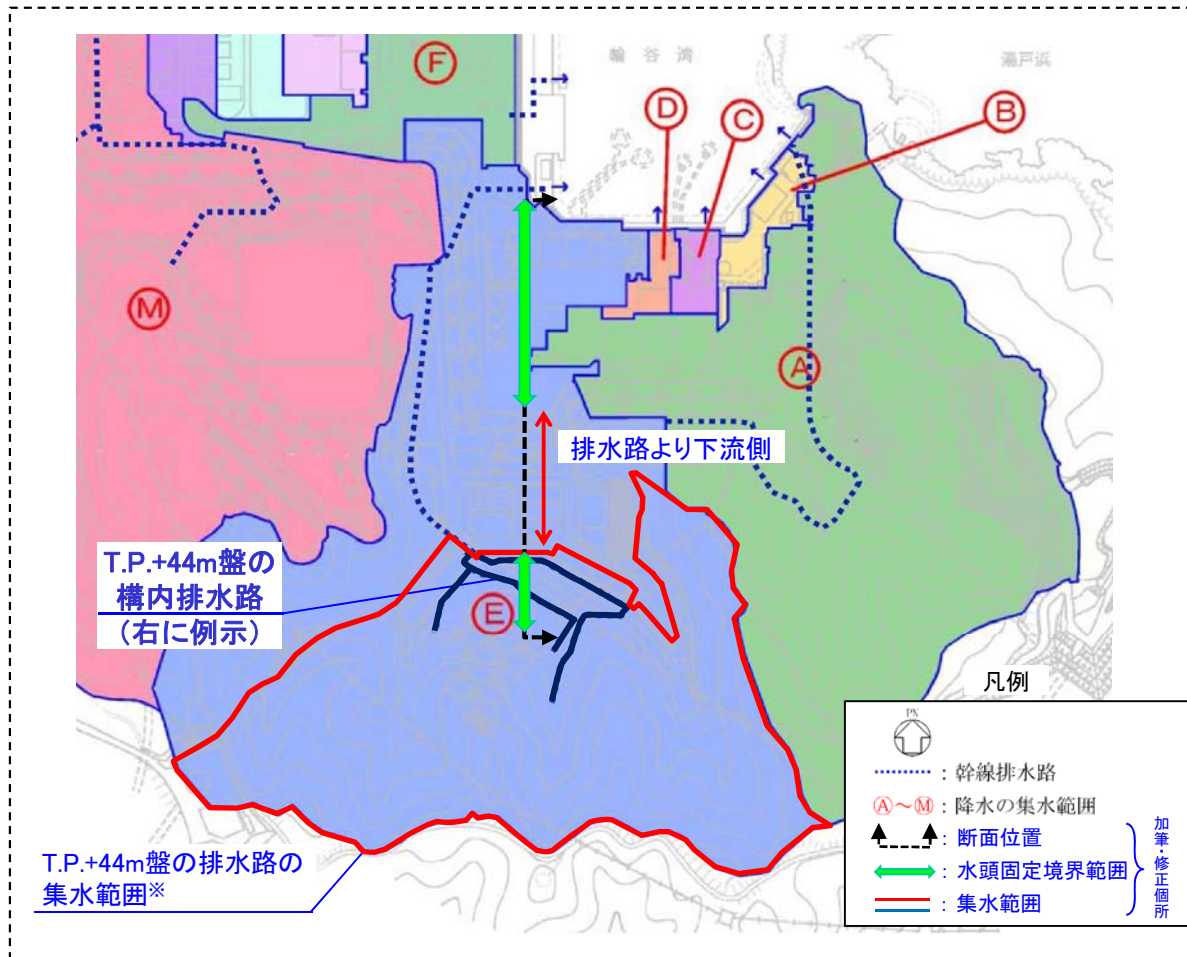
構内排水路位置図
