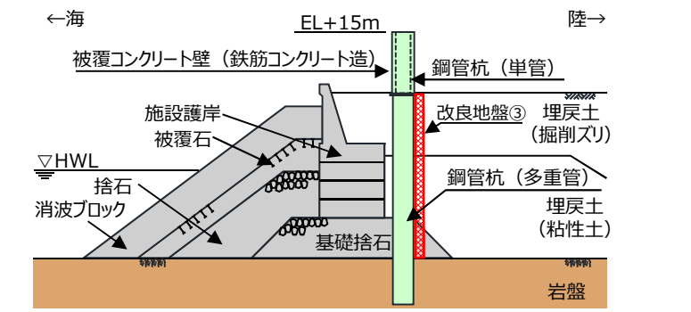
防波壁(多重鋼管杭式擁壁)断面図
