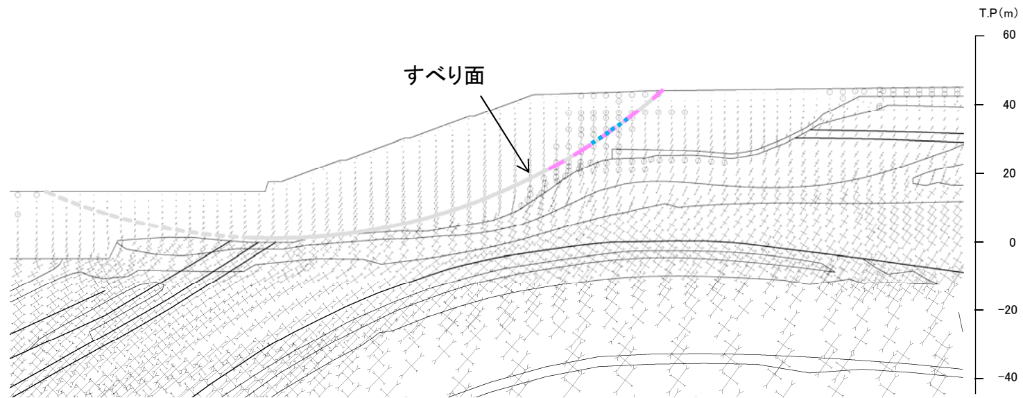
主応力分布図
