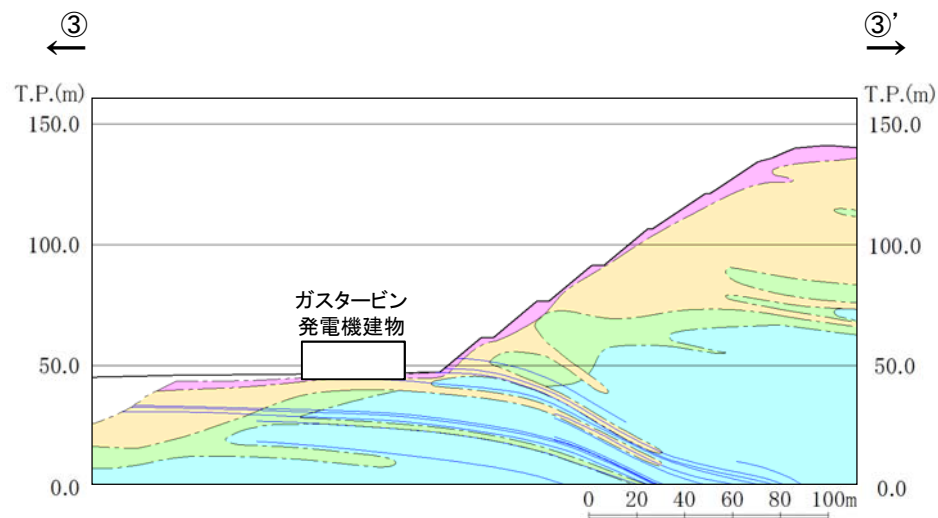
③-③' 断面図
