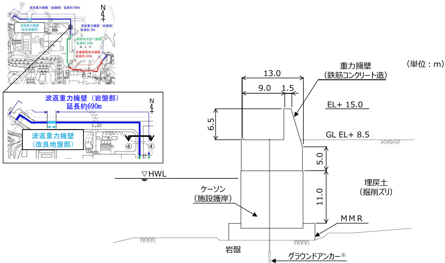
防波壁(波返重力擁壁)輪谷部(④-④断面) 断面図
