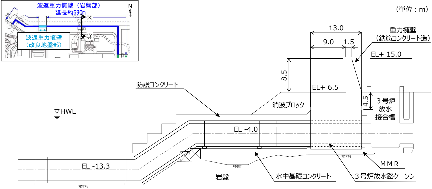
防波壁(波返重力擁壁)放水路貫通部(③-③断面) 断面図
