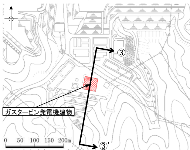
断面位置図
