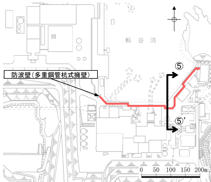
断面位置図
