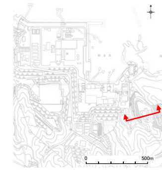
断面位置図
