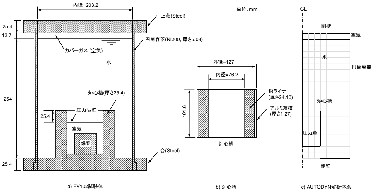
第 1.5.1 図 FV102 試験の試験体概要とAUTODYNの解析体系
