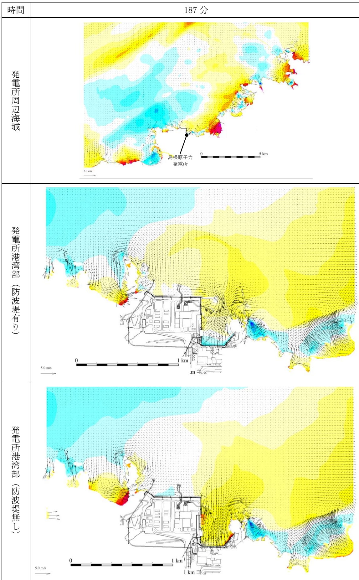
第 1 図 (175) 基準津波 1 の水位変動・流向ベクトル
