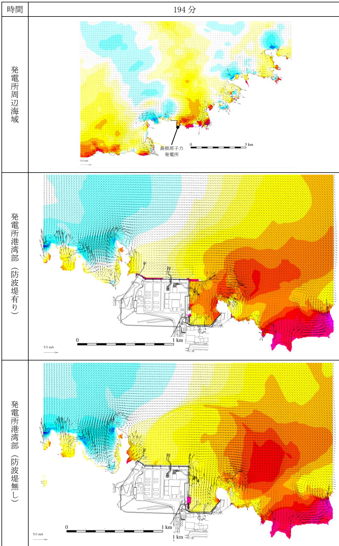
第 1 図(189) 基準津波 1 の水位変動・流向ベクトル
