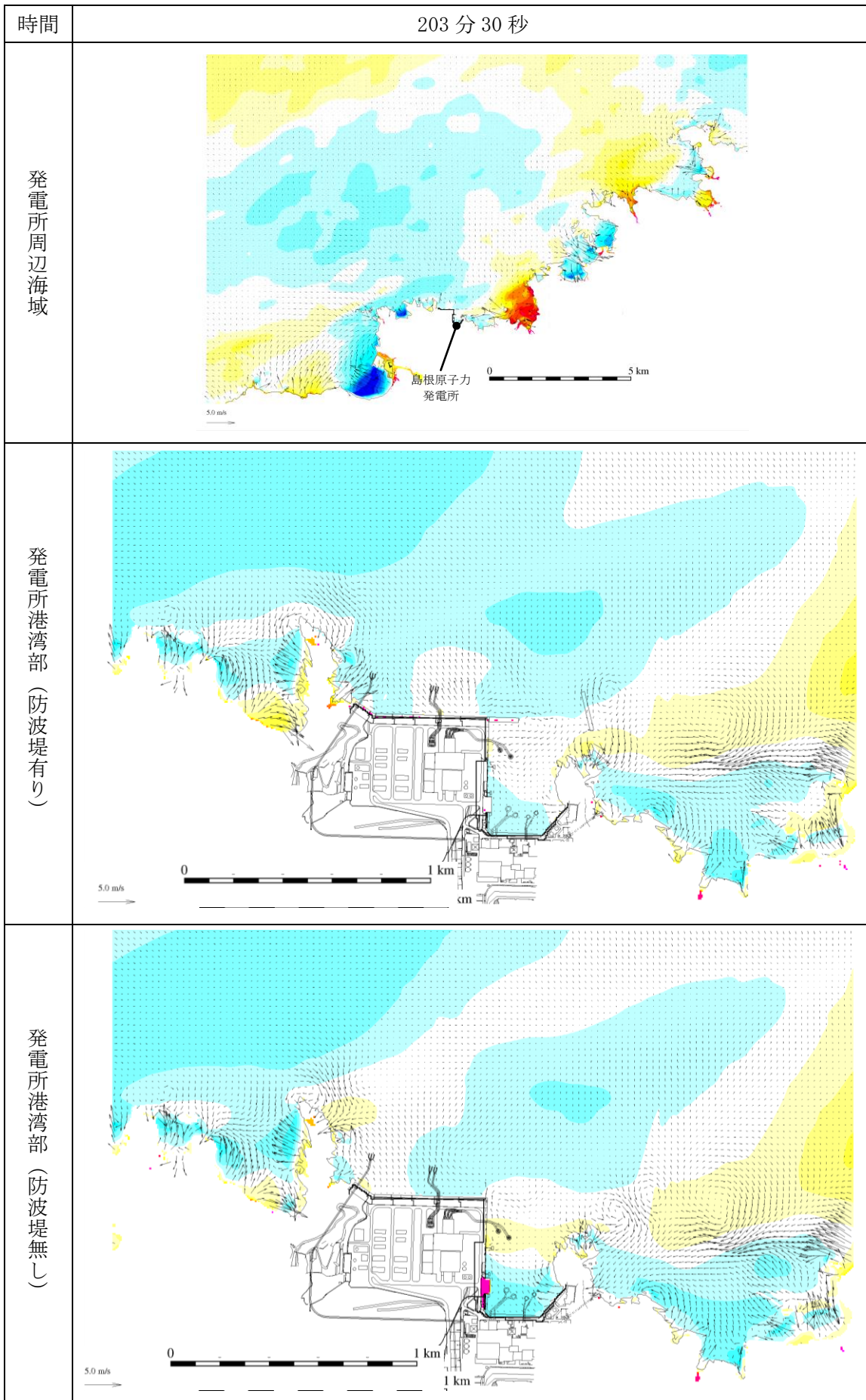
第 1 図 (208) 基準津波 1 の水位変動・流向ベクトル
