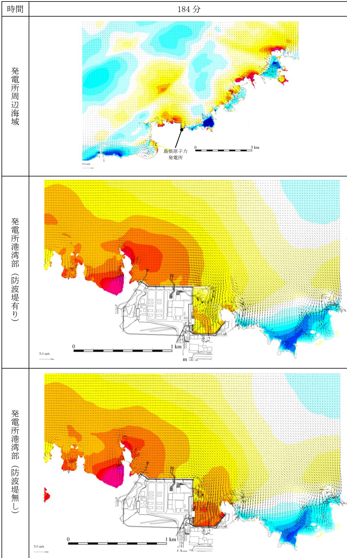
第 1 図(169) 基準津波 1 の水位変動・流向ベクトル
