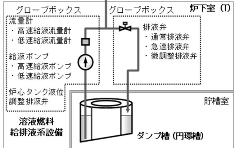
TRACYの主要系統構成
