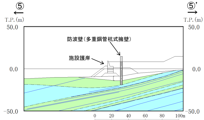
⑤-⑤' 断面図
