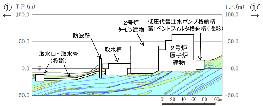
①-①' 断面図
