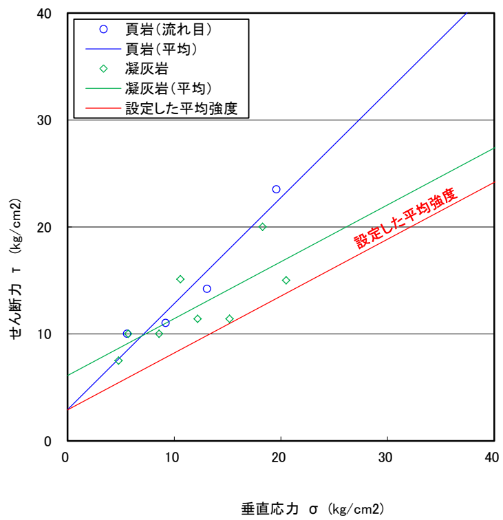
【設定方法例(C L 級頁岩と凝灰岩の互層:ピーク強度)】
