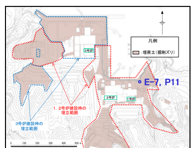
敷地平面図
