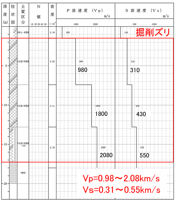
PS検層結果(3号炉エリア) ボーリングNo. E-3
