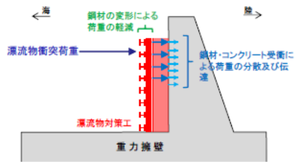
漂流物対策工における荷重図
