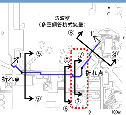
断面位置図
