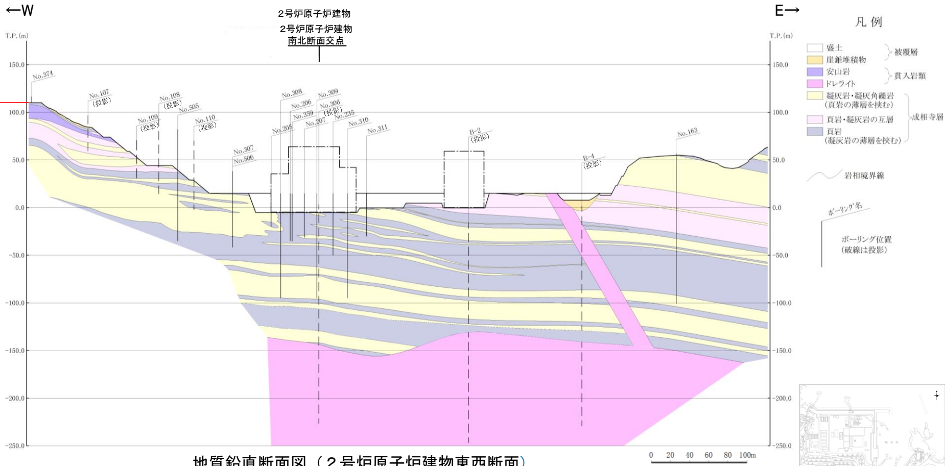
地質鉛直断面図 (2号炉原子炉建物東西断面)
