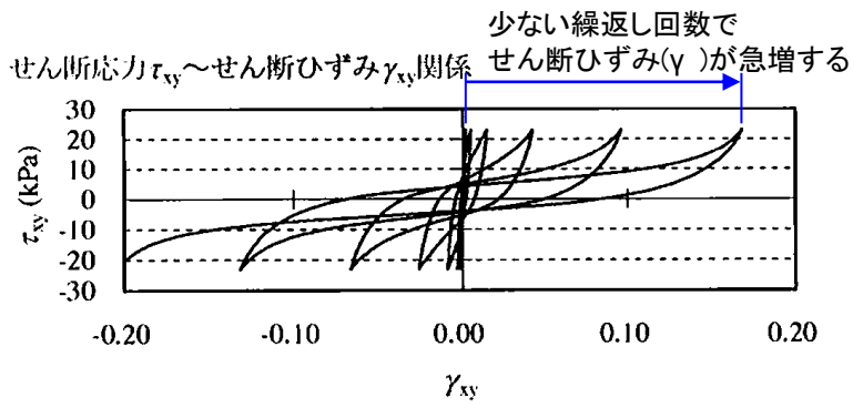
(a) せん断応力-せん断ひずみ関係
