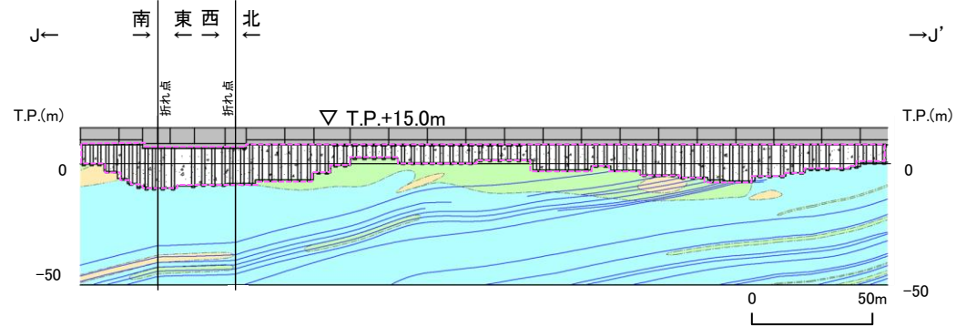
防波壁(鋼管杭式逆T擁壁) 縦断面図(岩級・シーム)
