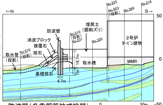
防波壁(多重鋼管杭式擁壁) I-4断面横断面図(岩級・シーム)
