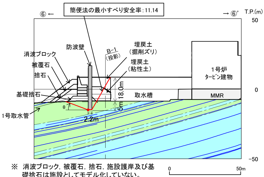
防波壁(多重鋼管杭式擁壁) ⑥-⑥'断面横断面図(岩級・シーム)
