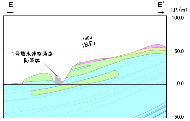
地質断面図(E-E'断面, 岩級・シーム) 0 50m
