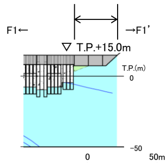
防波壁縦断面図(波返重力擁壁)
