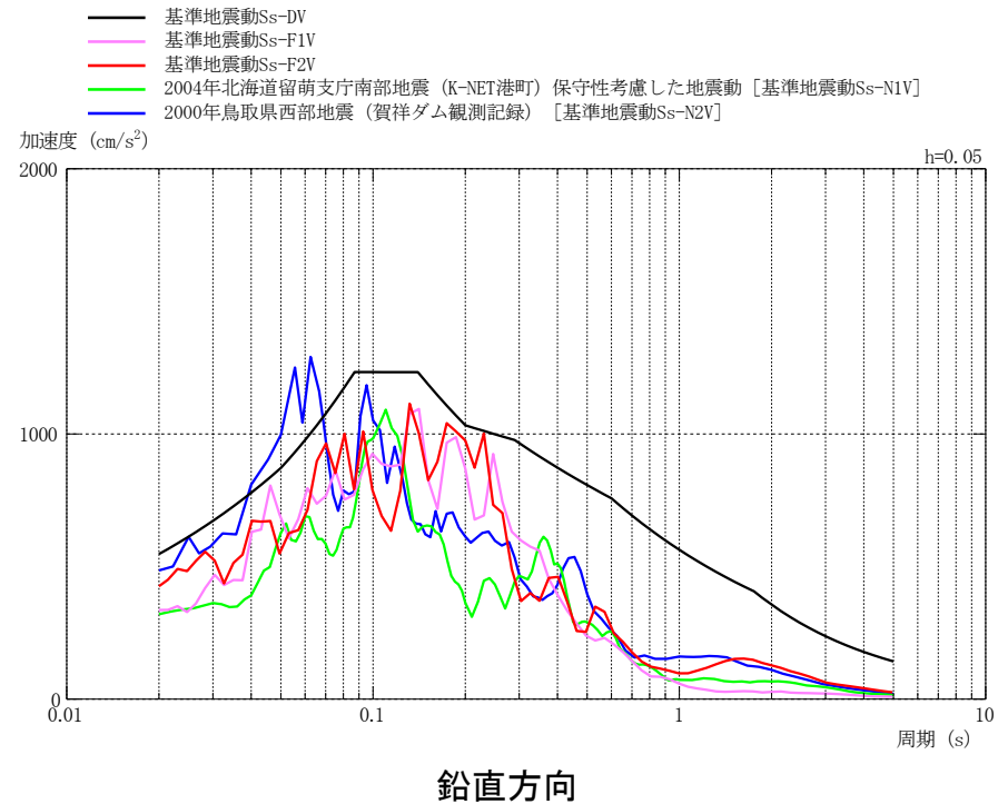
基準地震動の加速度応答スペクトル
