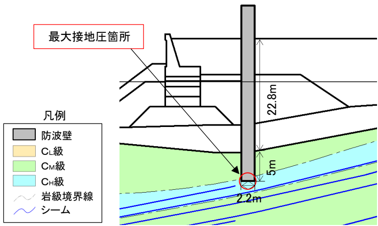
防波壁(多重鋼管杭式擁壁)
