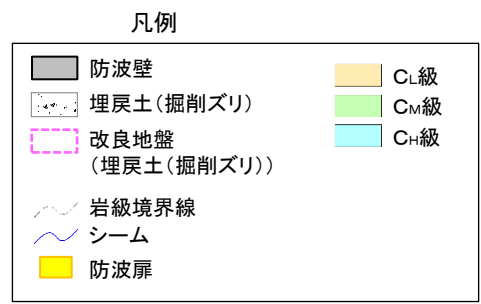
防波壁(鋼管杭式逆T擁壁)鉛直断面図 ※杭底面幅は、底面すべりにおける岩盤を通るすべり面の長さとしている。 当該施設では、杭先端のすべりを想定し、底面すべりの長さを杭間隔である6.6mとする。
