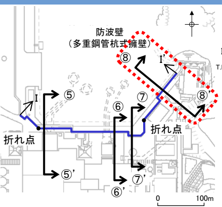
断面位置図
