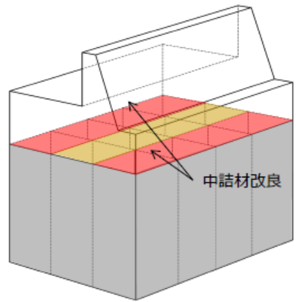
ケーソン(輪谷部)耐震補強対策工(例)
