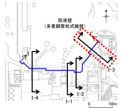
断面位置図
