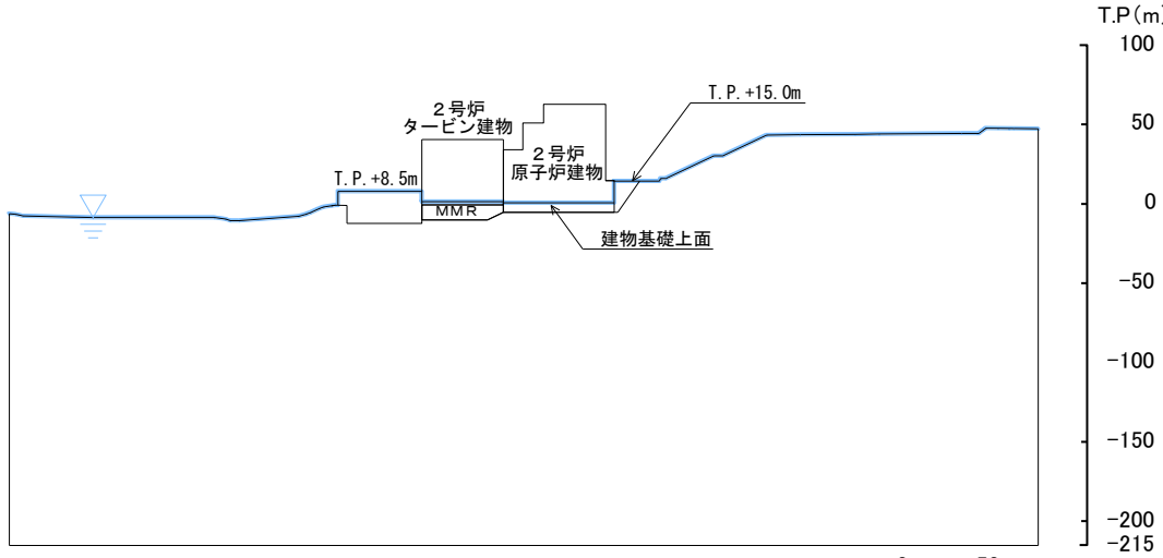
2号炉原子炉建物(南北) ①-①' 断面
