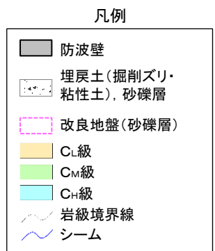
⑦-⑦'断面 簡便法の結果(液状化影響を考慮しない場合)
