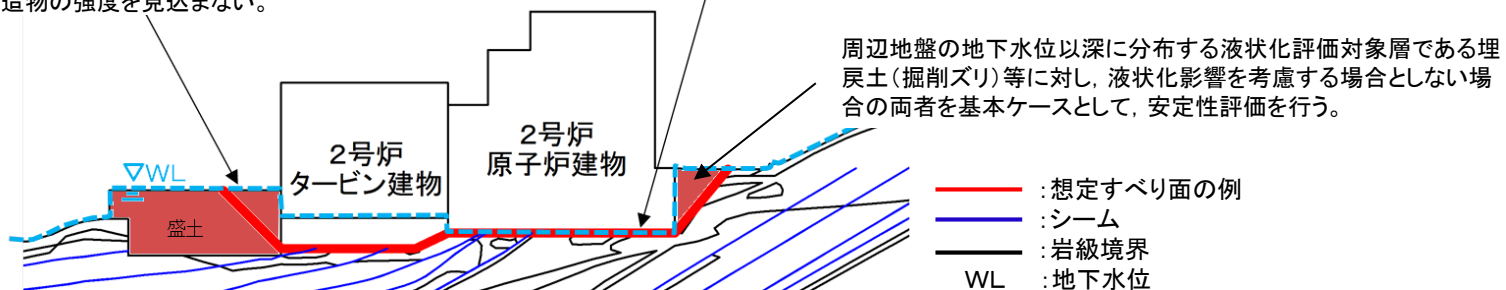
基礎地盤安定性評価における地下水位設定イメージ
