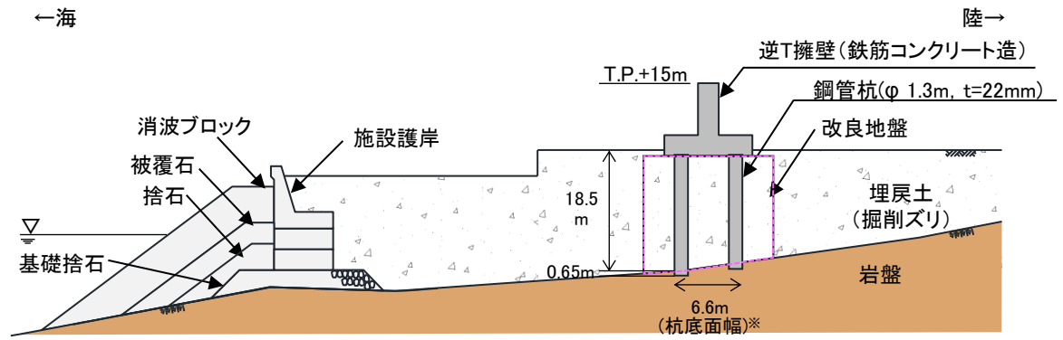
防波壁(鋼管杭式逆T擁壁)鉛直断面図 ※杭底面幅は、底面すべりにおける岩盤を通るすべり面の長さとしている。 当該施設では、杭先端のすべりを想定し、底面すべりの長さを杭間隔である6.6mとする。
