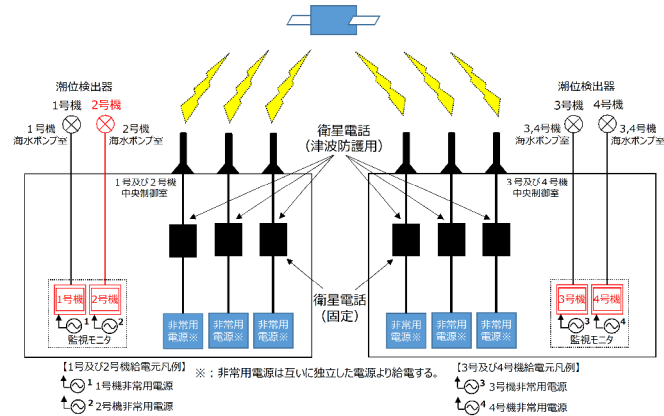
潮位観測システム（防護用）の概念図 （赤字部分が既認可と仕様又は設置場所が同じ設備）
