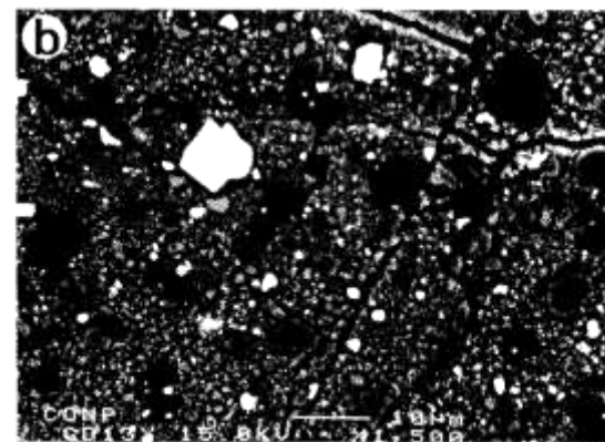
第7図 断層ガウジとシュードタキライト互層のSEM像(XX面)。a: 断層ガウジの組織にさらにシュードタキライトの層が含まれる。b: aの拡大。Pt: シュードタキライト。
