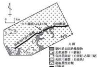
図-2 山田断層帯主部の南西部周辺の地質 地質は上村ほか 1) と黒田 2) を基に、一部改変した。山田断層帯を構成する断層帯の分布は地質調査院『地質調査年報』に基づく。図の範囲は図-1に示される。
