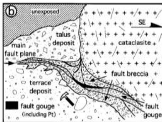
第3図 平林露頭(第1図のLoc. 1)の写角 (a) と詳細スケッチ (b)。断層破碎帯は花崗岩側に形成されたカタクレーサイト・岩塊角礫・断層ガウジおよびシュードタキライトから構成される。
