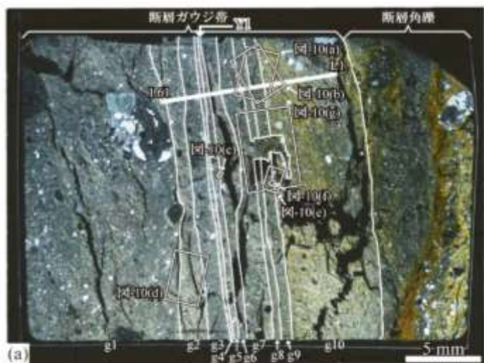
図-9 Y1 (a), Y5 (b) およびY6 (c) 沿いの薄片の全景写真
