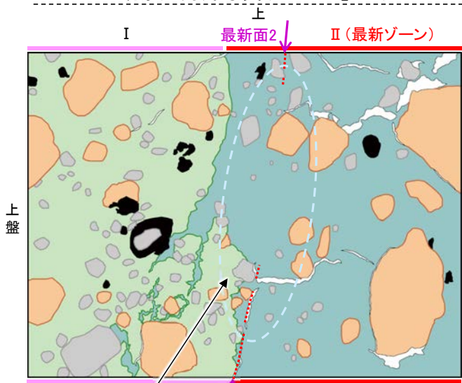
10mm 観察用薄片写真(H-6.6-1.71R)
