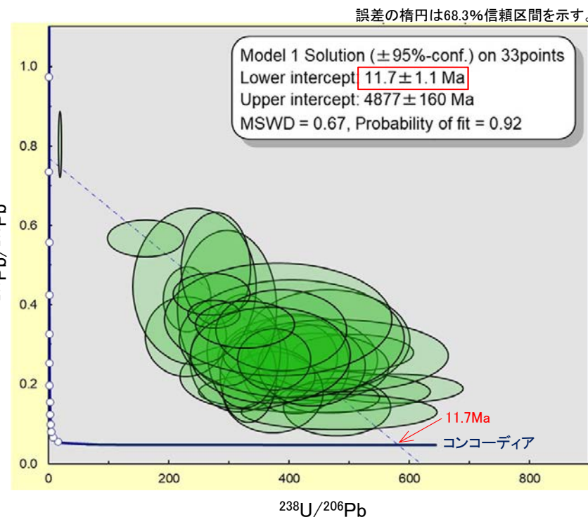
Total Pb Tera-Wasserburg コンコーディア図
