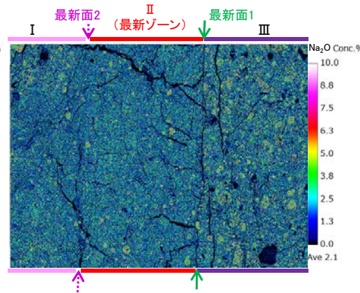
Na 2 O
