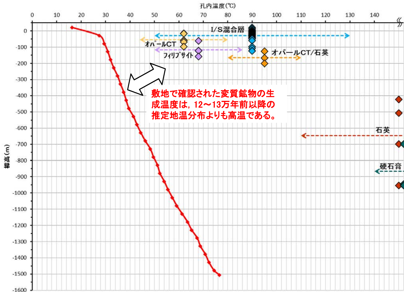
【変質鉱物の確認標高・生成温度と12~13万年前以降の敷地の地温分布の関係】
