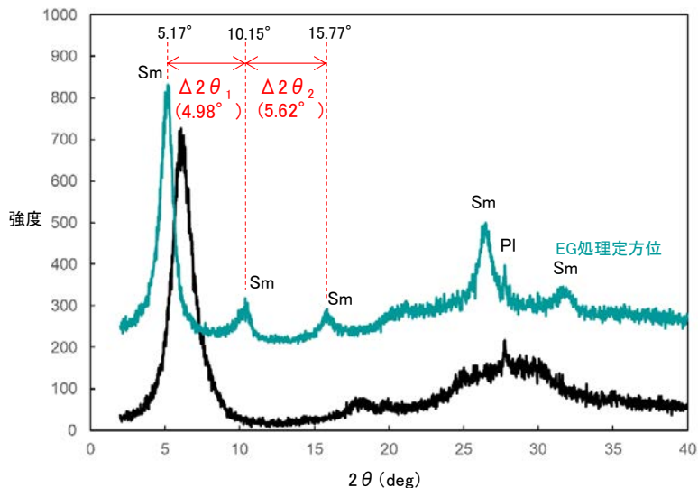
福浦灯台のX線回折チャート
