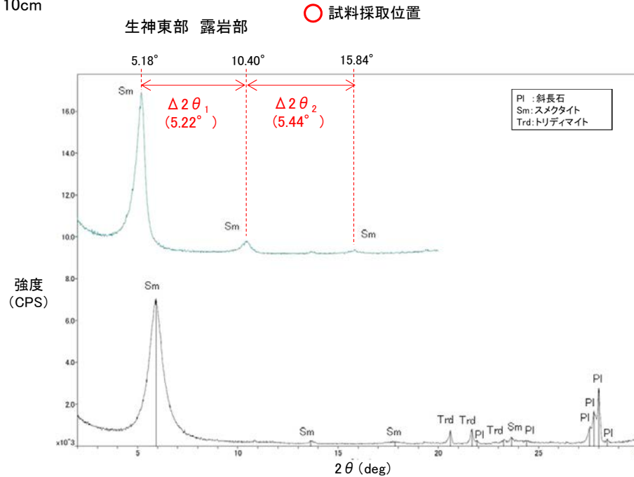
X線回折チャート
