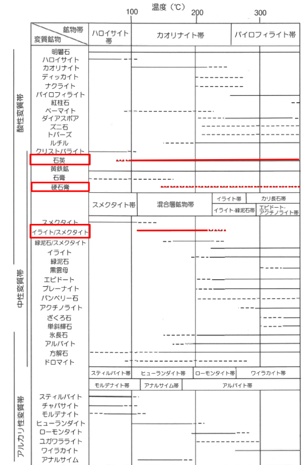
各変質帯に特徴的な鉱物とそれらの概略の生成温度 (井上(2003)に一部加筆)
