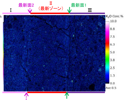
K 2 O
