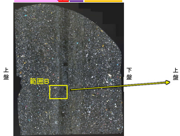
10mm 観察用薄片写真(H-6.6-1.71R)
