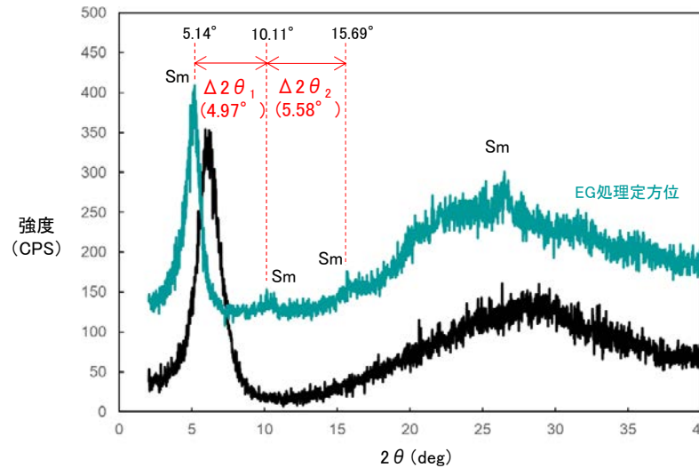
X線回折チャート
