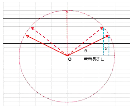
図 2.1 竜巻の発生と移動の概念図
