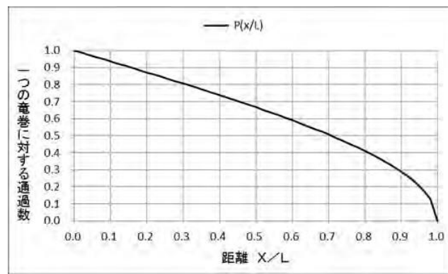
図 2.2 帯状領域での竜巻の通過数
