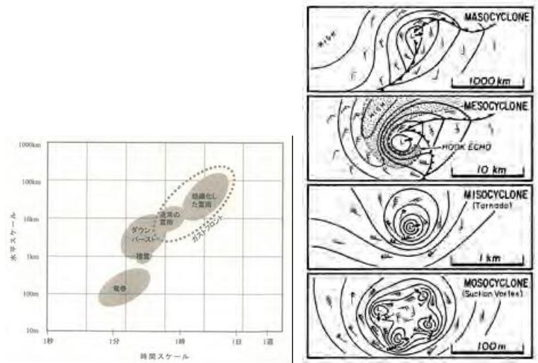
図2 竜巻発生時の渦の多重構造 (Fujita 1981)
