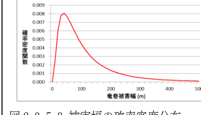
図2.3.5.3 被害幅の確率密度分布
