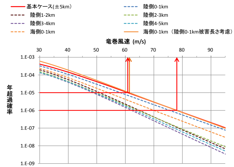
第 2.2.2.2-8 図 竜巻最大風速のハザード曲線
