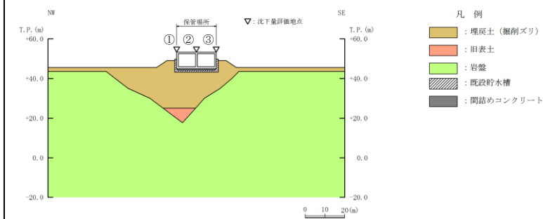
断面図 (短辺方向)
