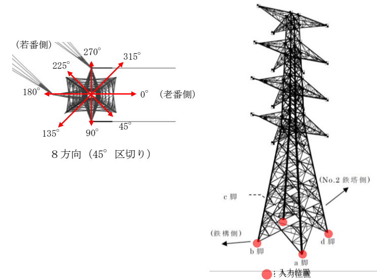
第12図 地震動の入力方向及び位置
