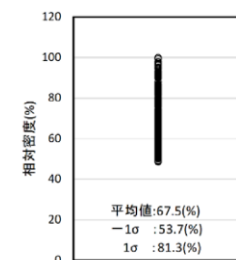
第5図 As 層 (砂層) の相対密度
