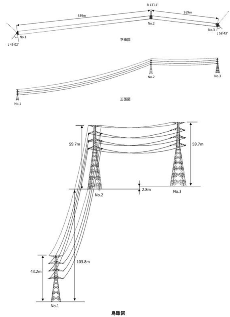
第 11 図 220kV 第二島根原子力幹線 No. 2 鉄塔を 主とした連成系モデル
