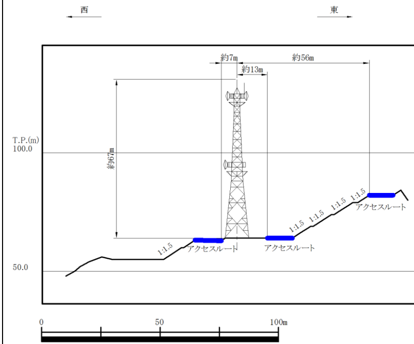
⑨ 通信用無線鉄塔
