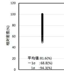
第6図 Ag1層（砂礫層）の相対密度
