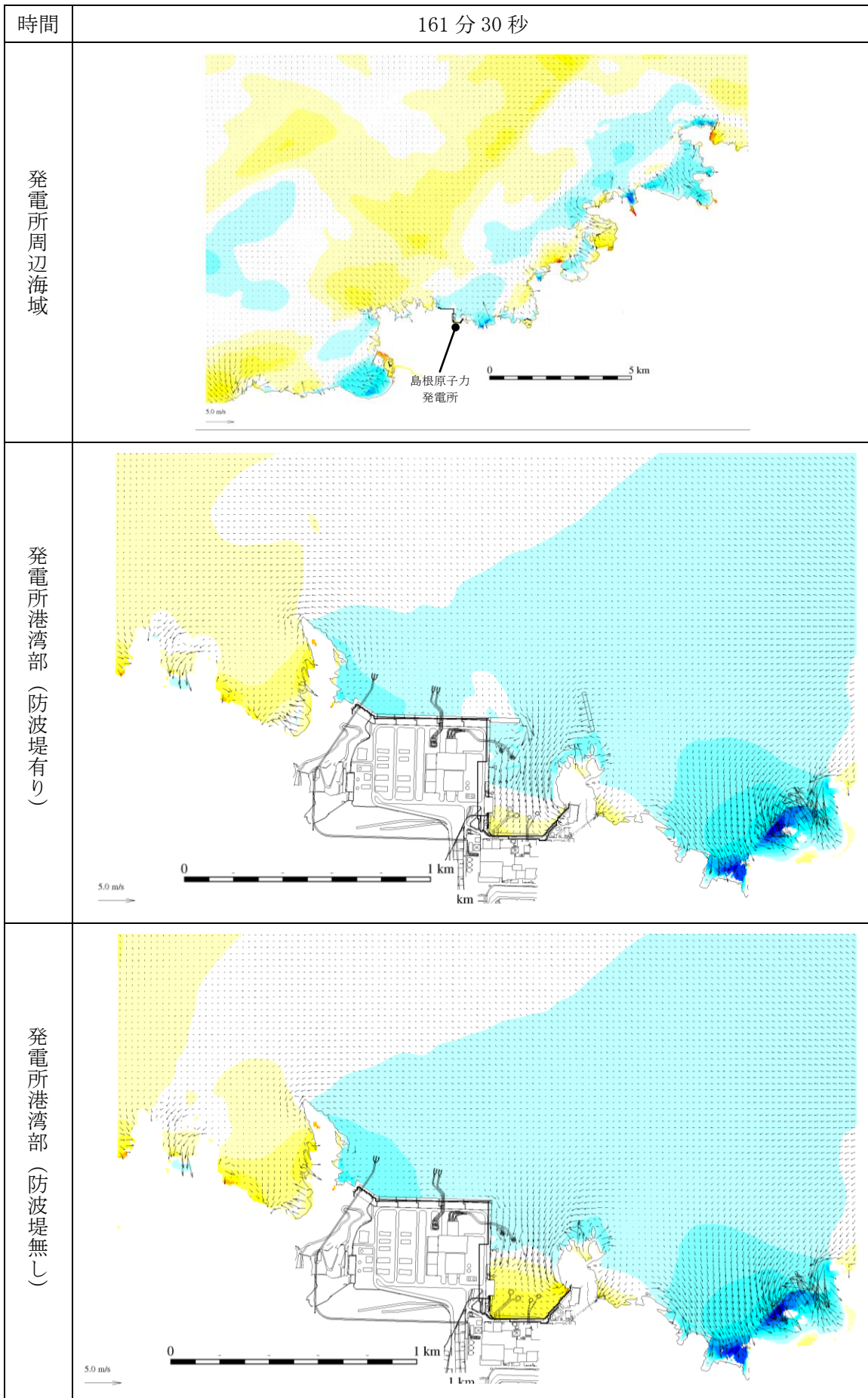
第 1 図(124) 基準津波 1 の水位変動・流向ベクトル
