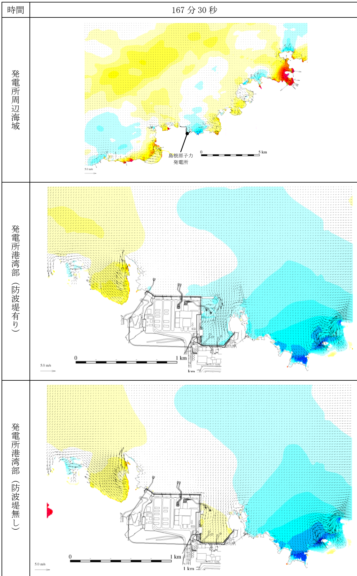
第 1 図 (136) 基準津波 1 の水位変動・流向ベクトル
