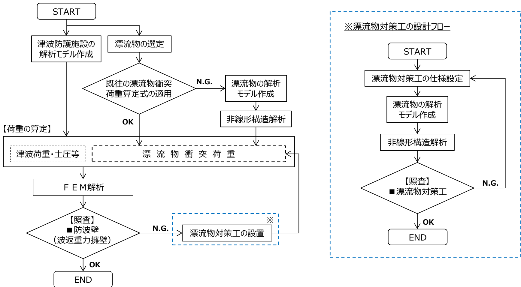
防波壁（波返重力擁壁）における津波防護施設の設計フロー（例）
