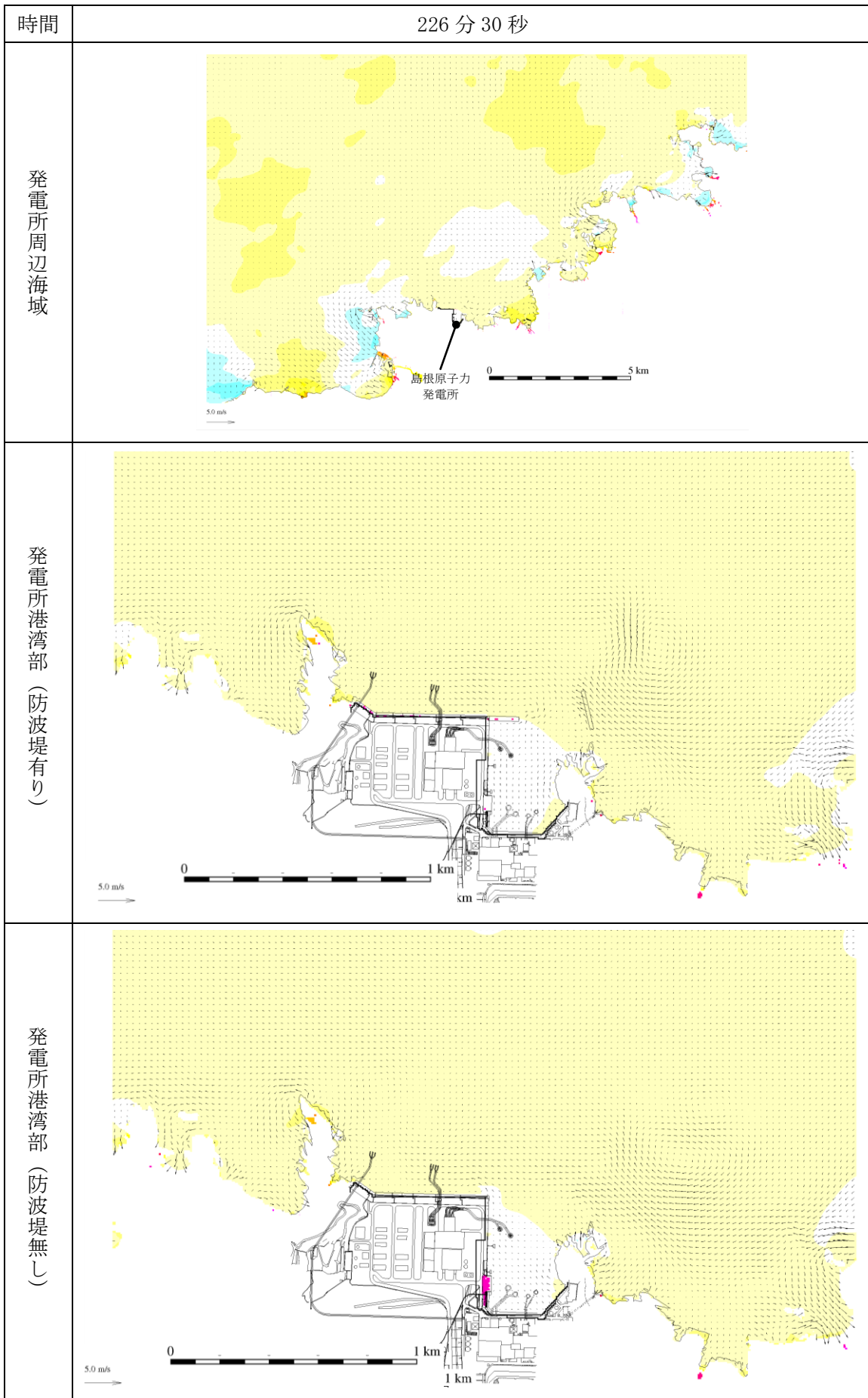
第 1 図 (254) 基準津波 1 の水位変動・流向ベクトル
