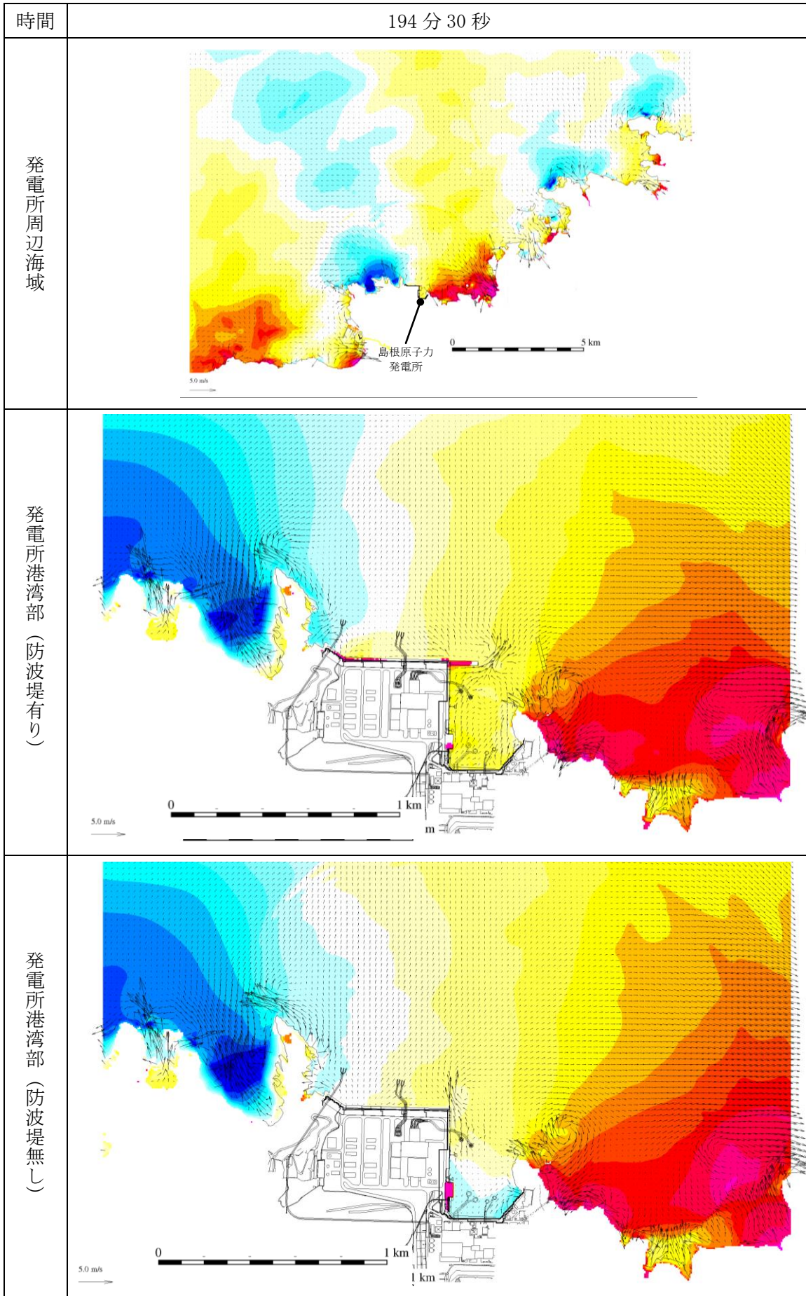
第 1 図(190) 基準津波 1 の水位変動・流向ベクトル
