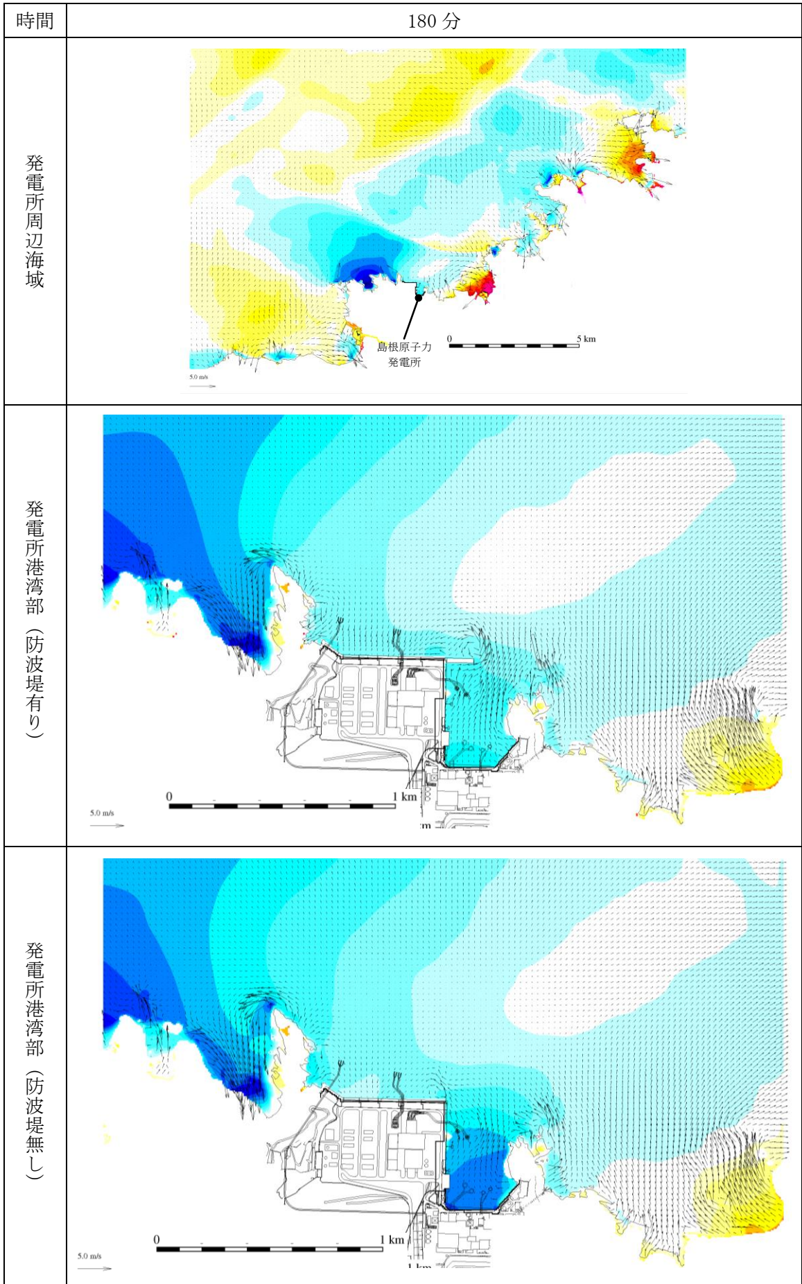
第 1 図(161) 基準津波 1 の水位変動・流向ベクトル
