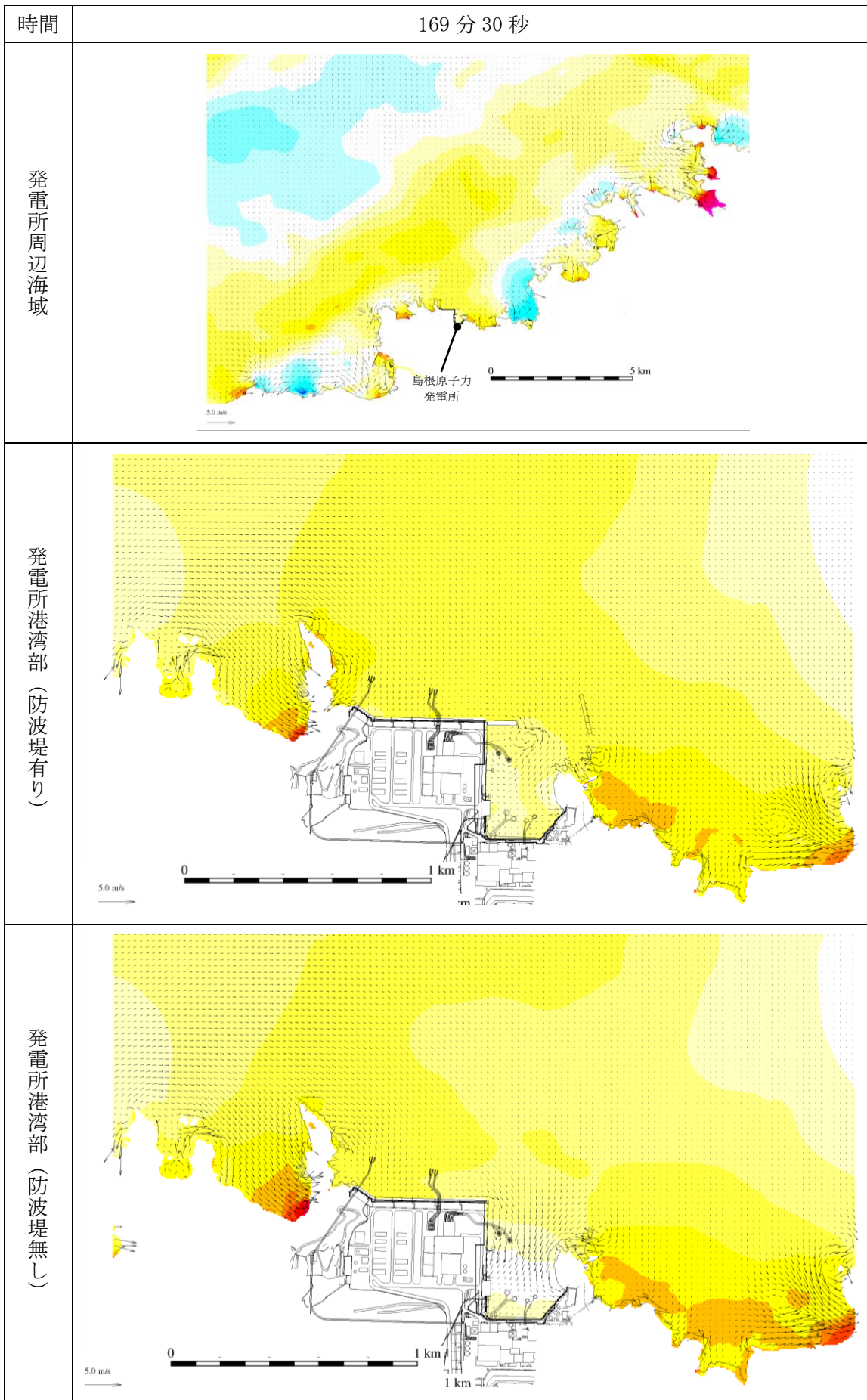
第 1 図(140) 基準津波 1 の水位変動・流向ベクトル
