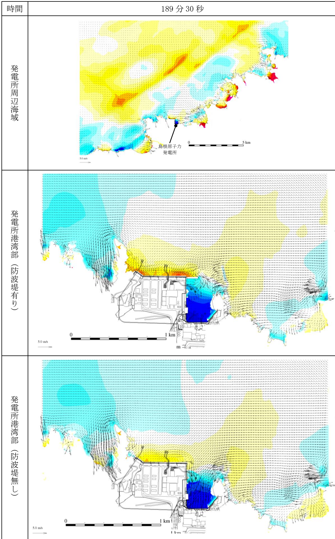
第 1 図(180) 基準津波 1 の水位変動・流向ベクトル
