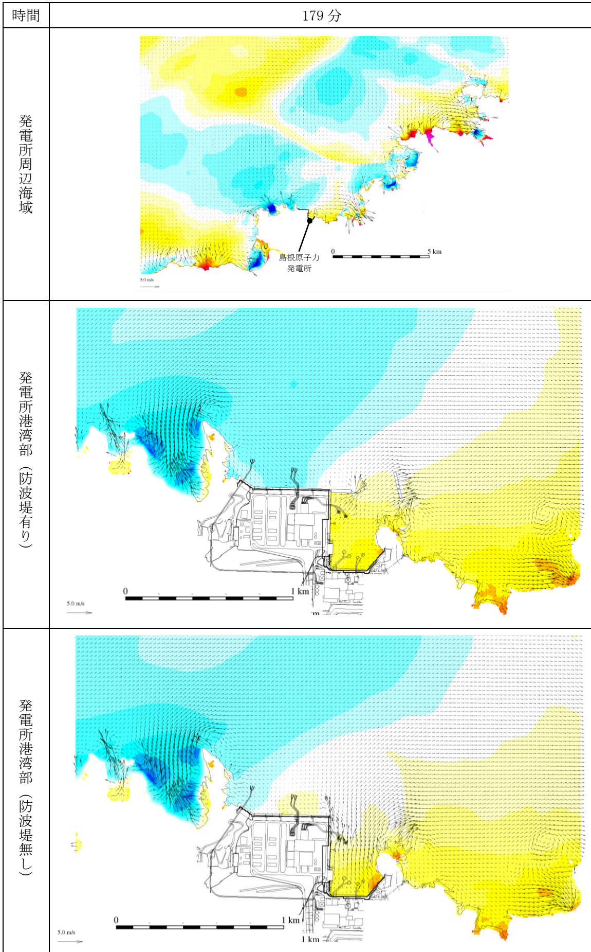
第 1 図(159) 基準津波 1 の水位変動・流向ベクトル
