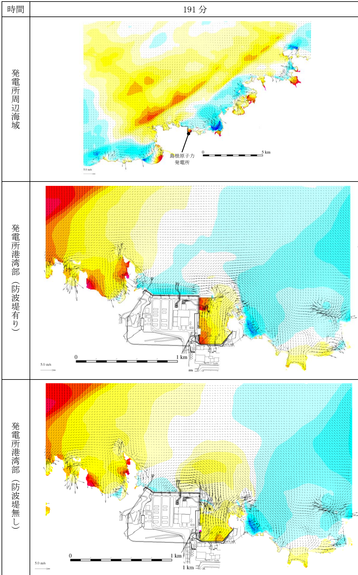
第 1 図(183) 基準津波 1 の水位変動・流向ベクトル
