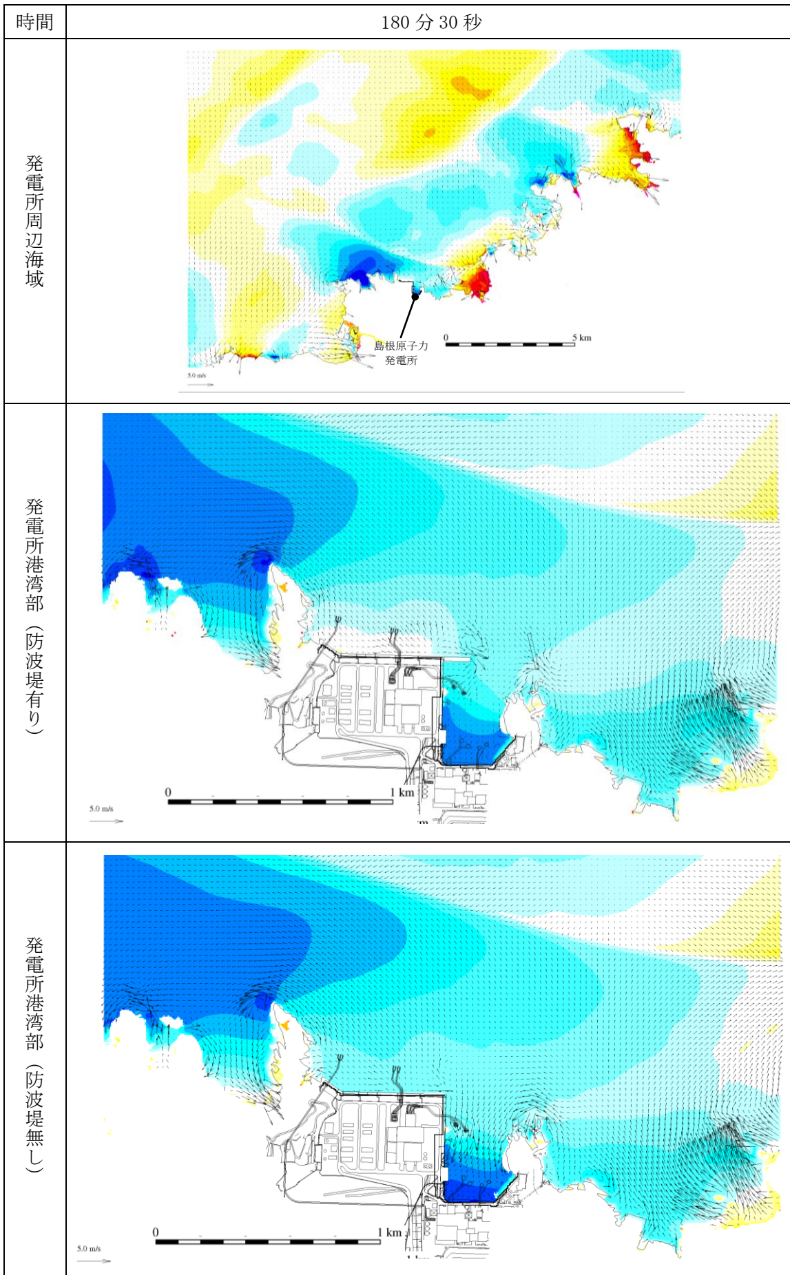
第 1 図(162) 基準津波 1 の水位変動・流向ベクトル
