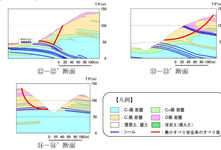
第 4-12 図 周辺斜面の安定性評価結果 (2 / 4)
