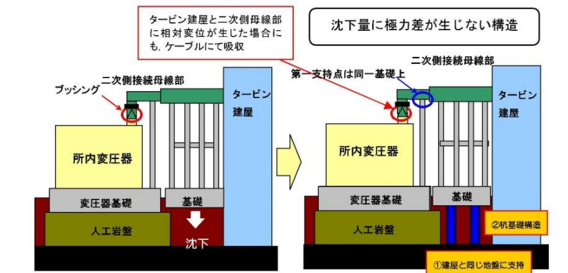
第2図 変圧器火災の対策(7号炉所内変圧器)
