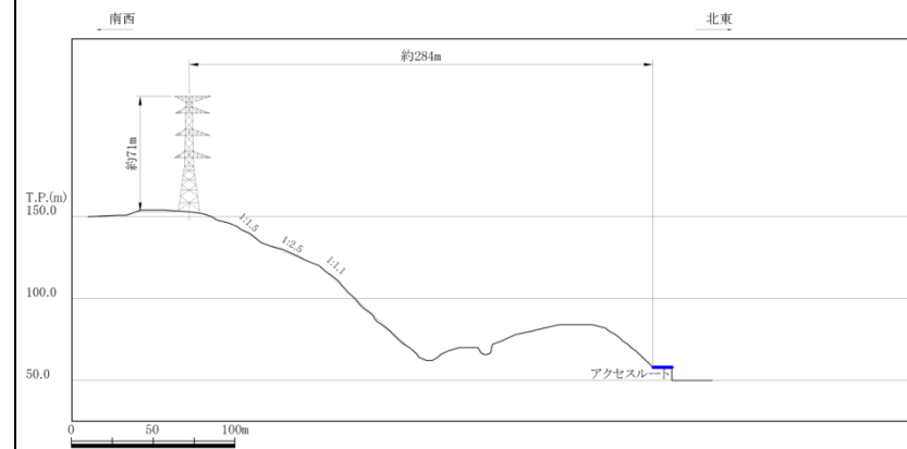
①-1 500kV 島根原子力幹線 No. 3 鉄塔(傾斜方向)
