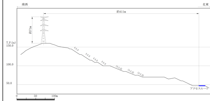
⑦-1 500kV 島根原子力幹線 No. 2 鉄塔 (傾斜方向)
