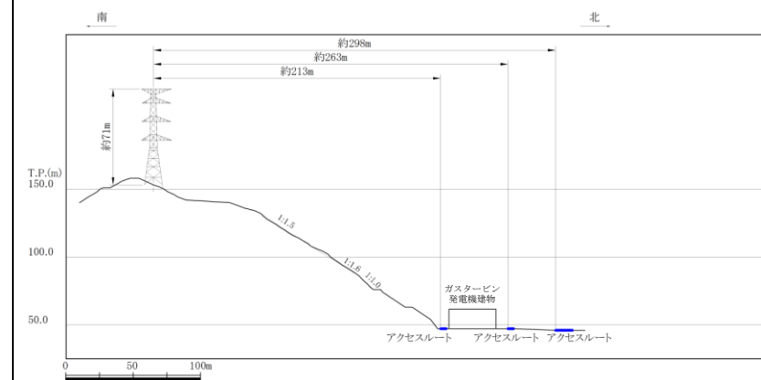
①-2 500kV 島根原子力幹線 No. 3 鉄塔 (アクセスルート最短(北側))
