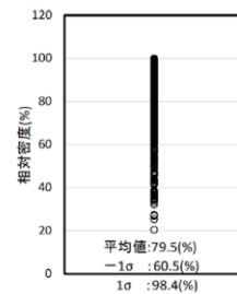
第4図 Ag2 層 (砂礫層) の相対密度
