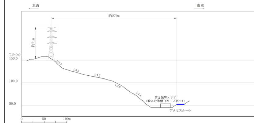
①-3 500kV 島根原子力幹線 No. 3 鉄塔 (アクセスルート最短(北西側))
