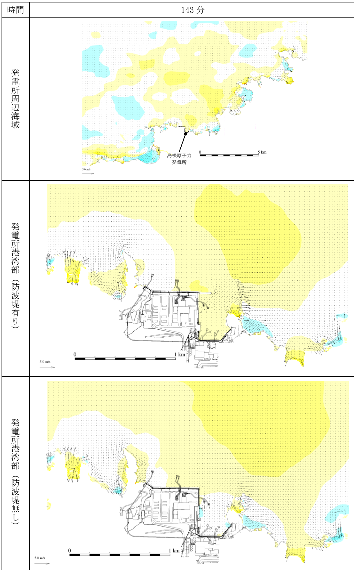
第 1 図(87) 基準津波 1 の水位変動・流向ベクトル
