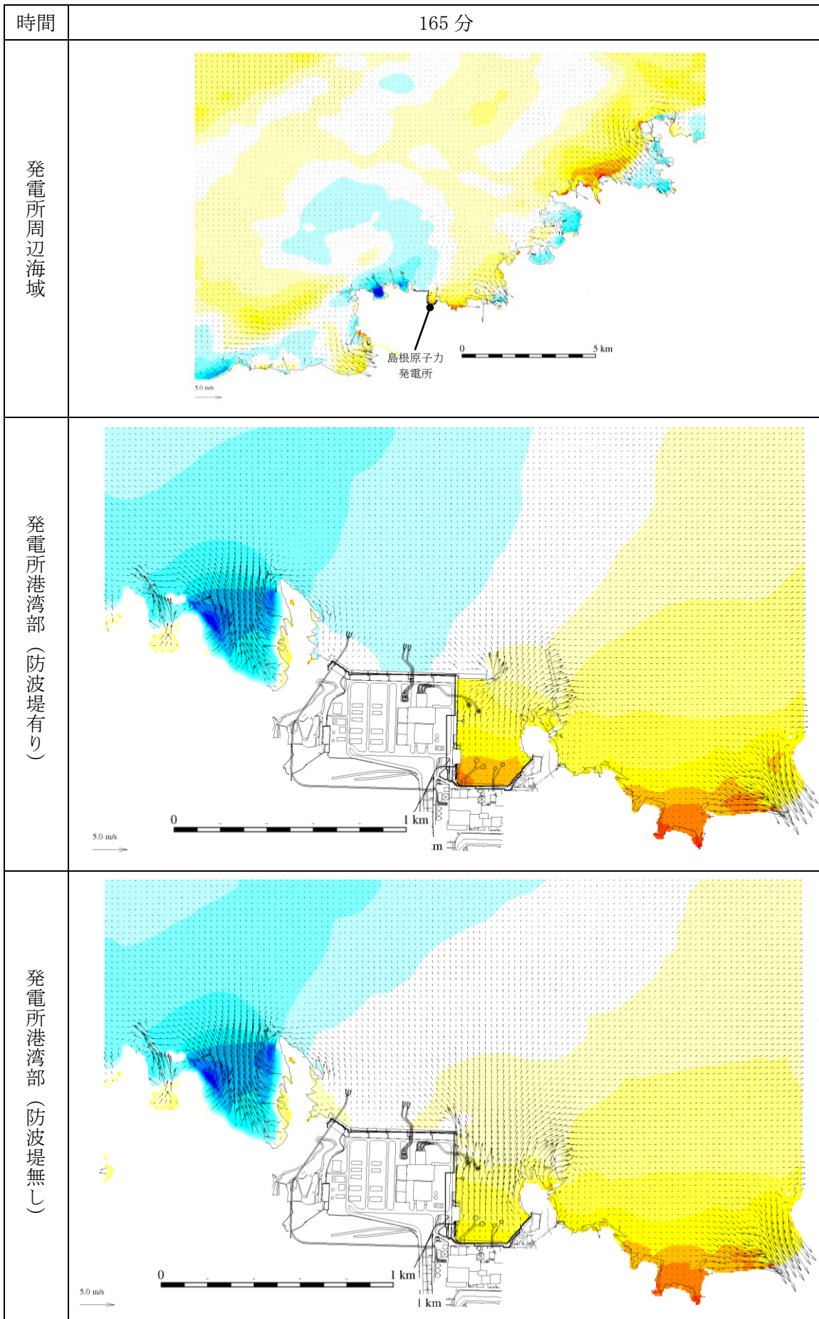
第 1 図(131) 基準津波 1 の水位変動・流向ベクトル
