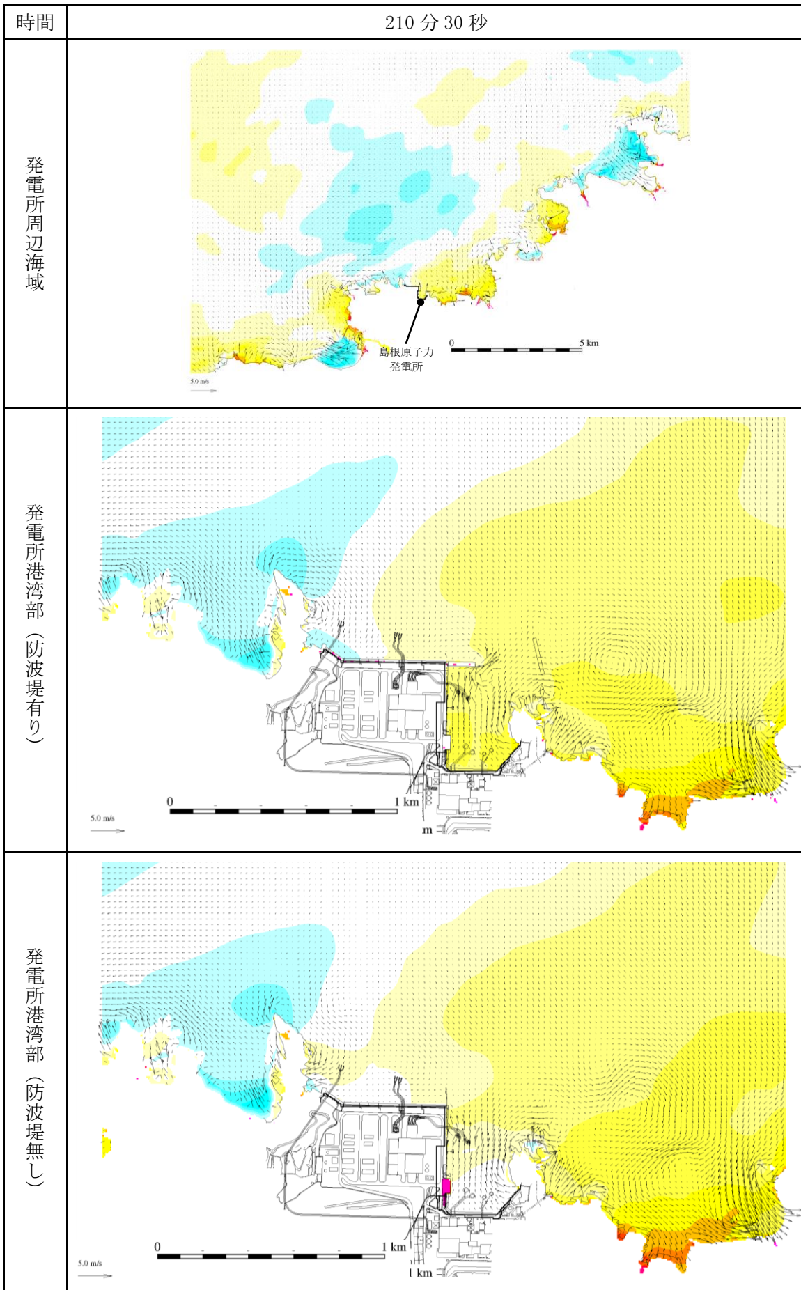
第 1 図 (222) 基準津波 1 の水位変動・流向ベクトル
