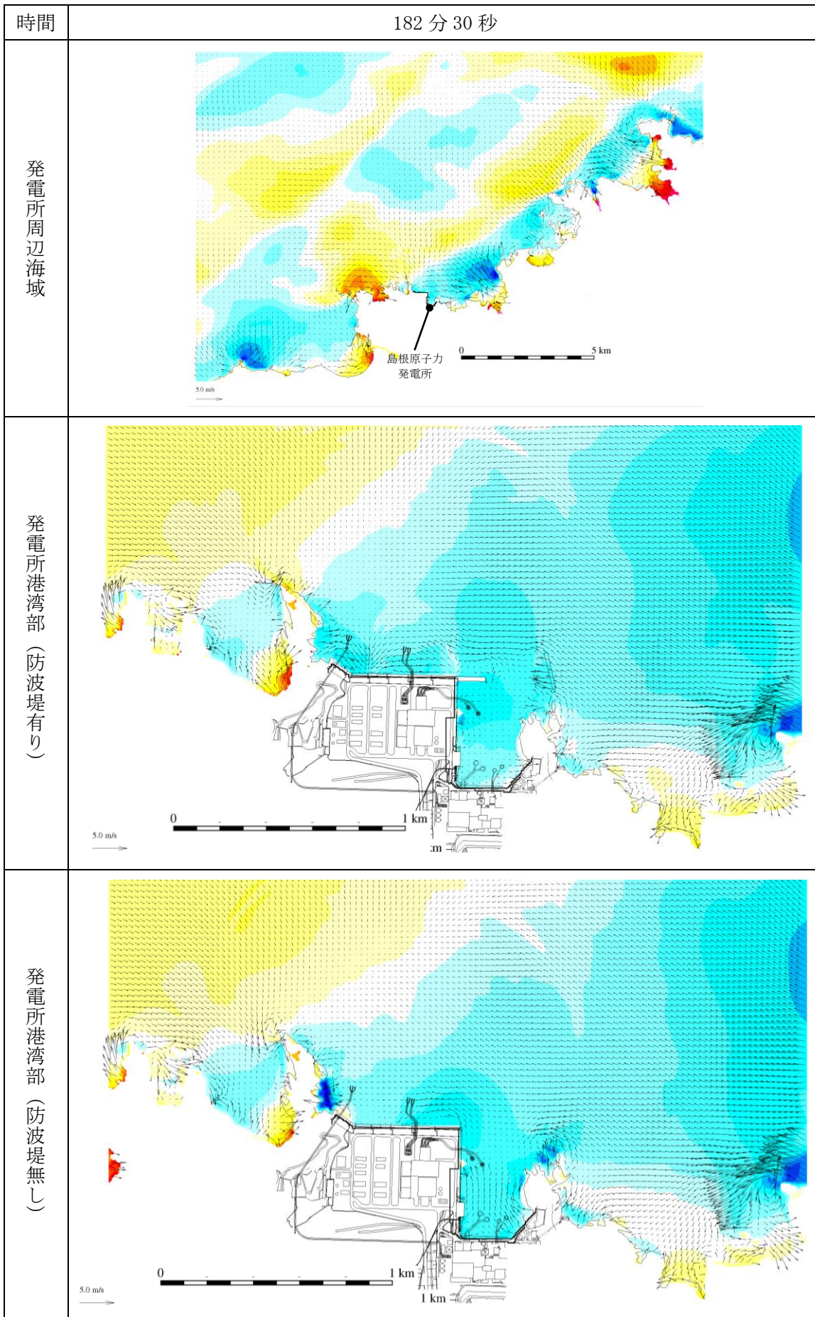
第 1 図(166) 基準津波 1 の水位変動・流向ベクトル
