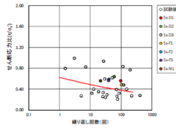
第5.4-10図 累積損傷度理論に基づく評価結果 (D-1)
