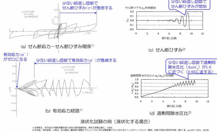
【液状化試験のイメージ (1)】
