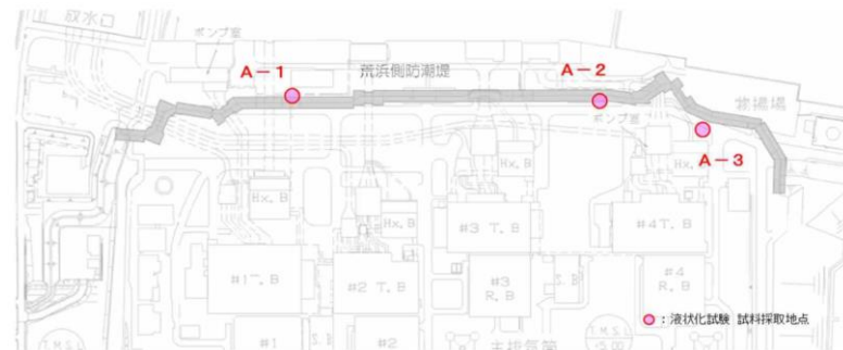
(a) 平面図
