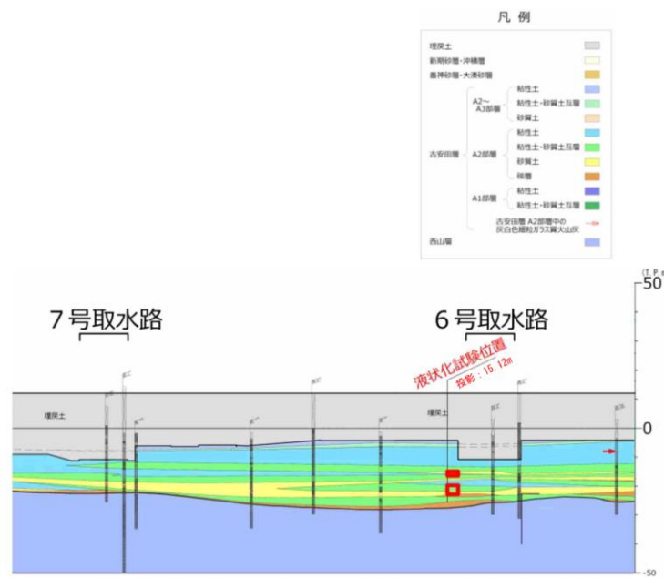
(b) 断面図
