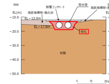
取水管
