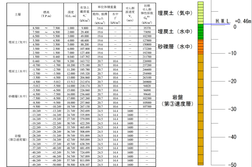
地盤物性値
