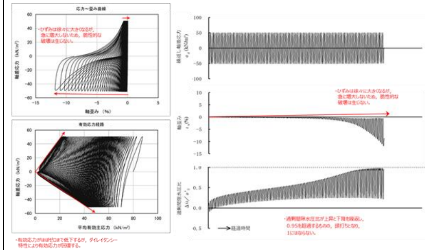
第3-2-18 図 液状化試験結果の例 (E地点の埋戻土(掘削ズリ))
