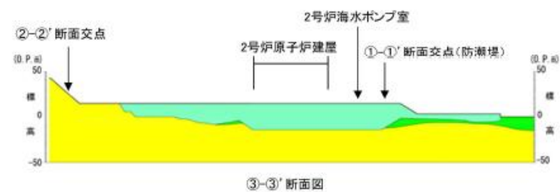
③-③' 断面図
