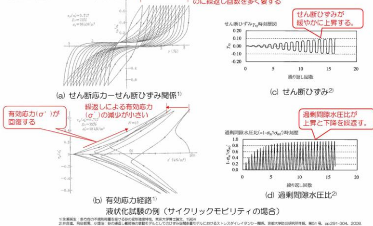
【液状化試験のイメージ (2)】
