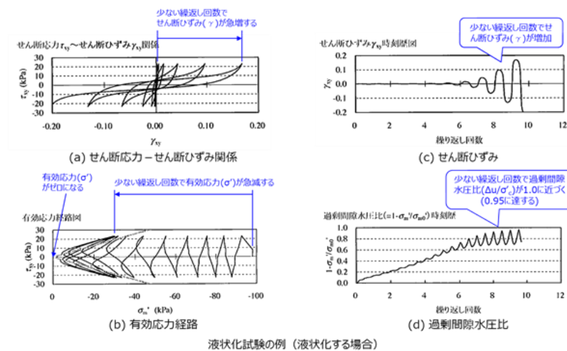
第3-2-5 図 緩い砂の液状化試験結果
