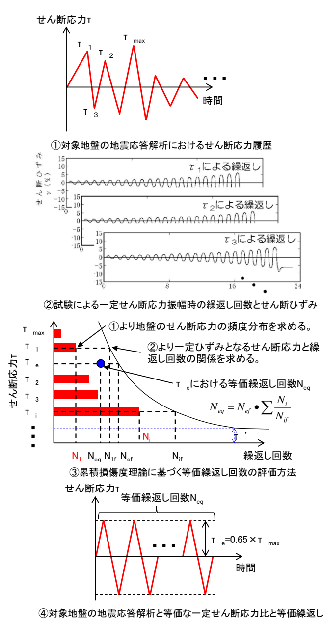
第3-3-2 図 累積損傷度理論に基づく等価繰返し回数の評価方法
