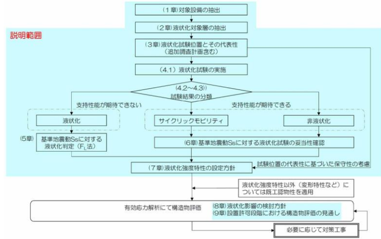
第11-1-1 図 液状化評価の流れ
