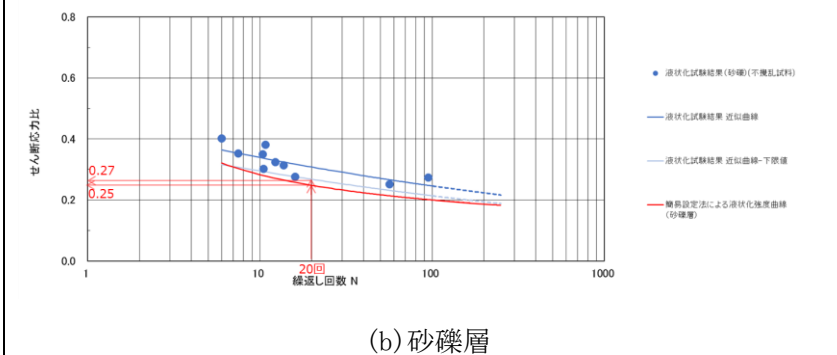
第3-5-1 図 簡易設定法及び液状化試験結果による液状化強度曲線の比較
