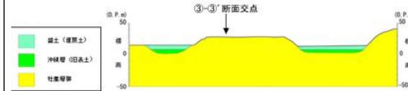
②-②' 断面図
