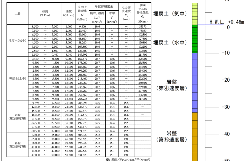
地盤物性値
