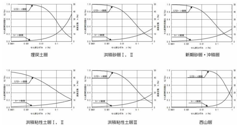
(c) せん断剛性及び減衰のひずみ依存性 (A-2 及びA-3 地点) 第11-6-3 図 解析用物性値及び解析モデル
