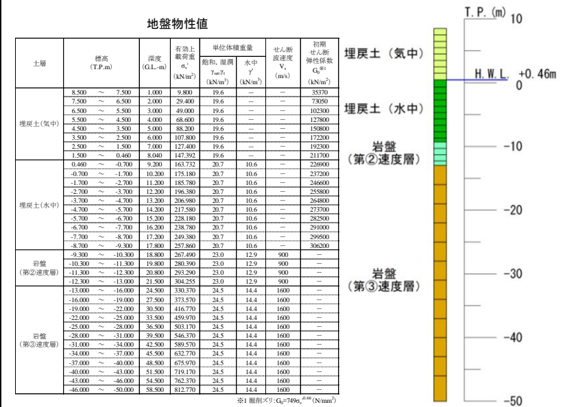
(f) 基本物性 (比較地点⑥)
