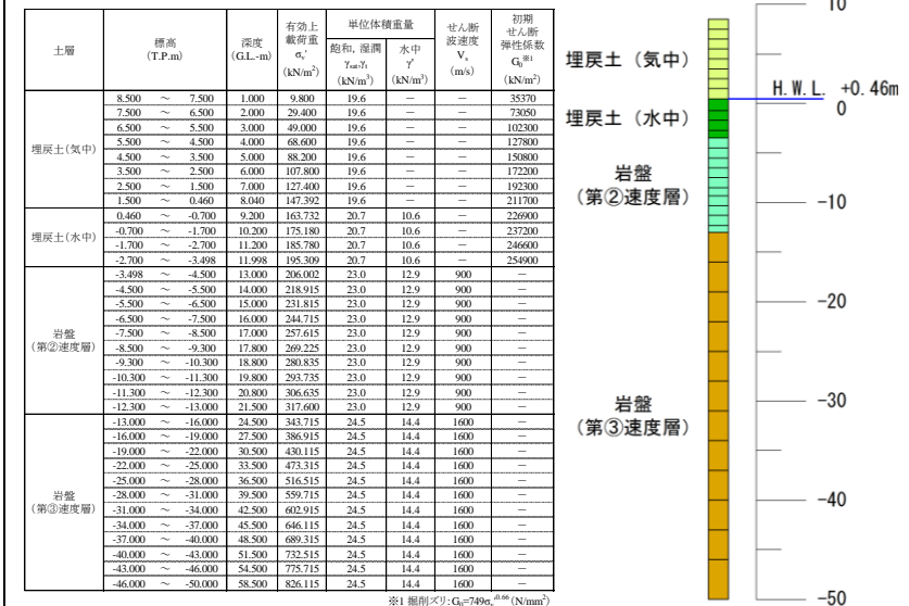
地盤物性値
