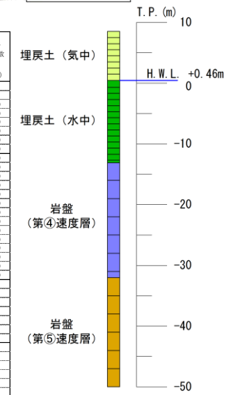
(c) 基本物性 (比較地点③) 第3-3-5 図 解析用物性値及び解析モデル
