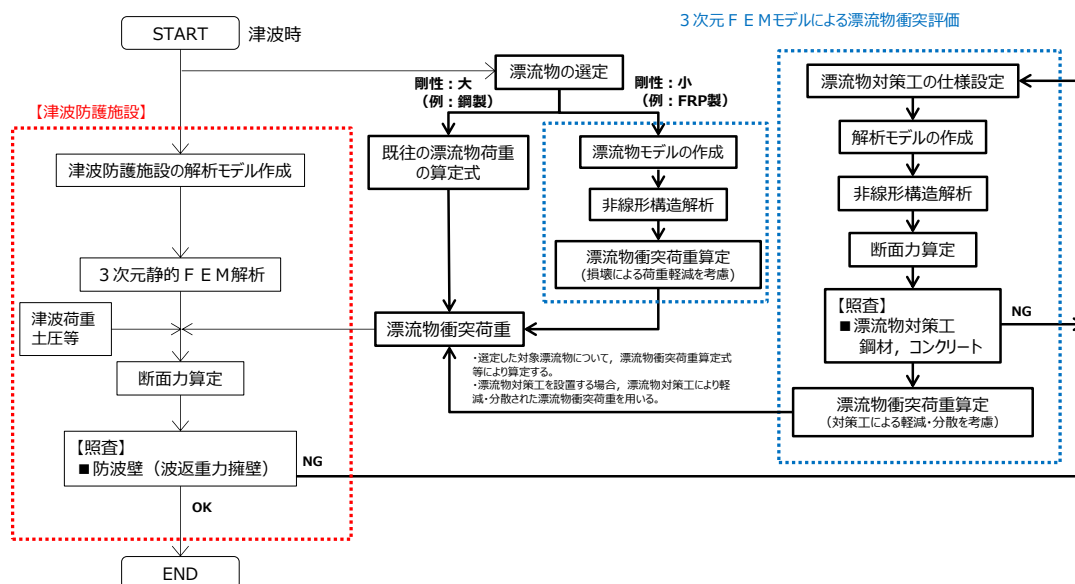
図-26 防波壁（波返重力擁壁）における津波防護施設的设计フロー（例）
