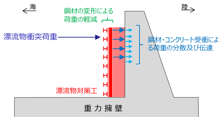
図－25 防波壁（波返重力擁壁）の漂流物対策工における荷重図
