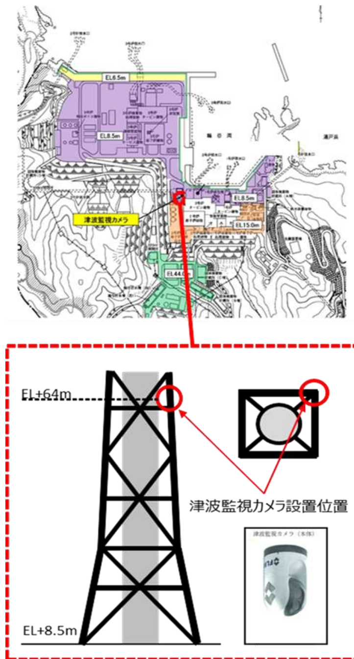
第4.3-2図 津波監視カメラ設置位置
