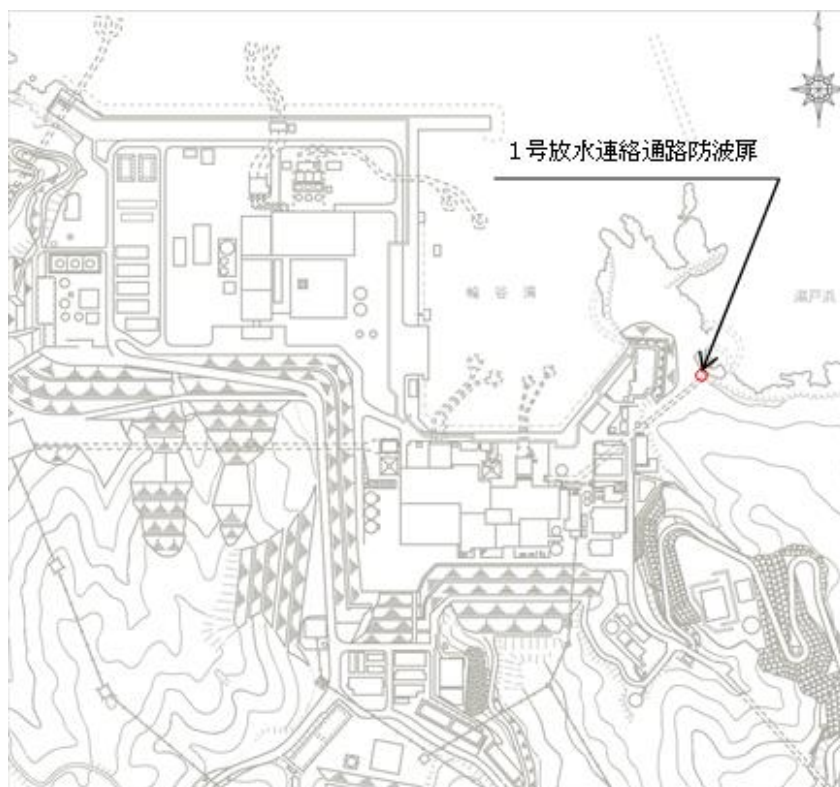
第 4.1-8 図 1号放水連絡通路防波扉配置図
