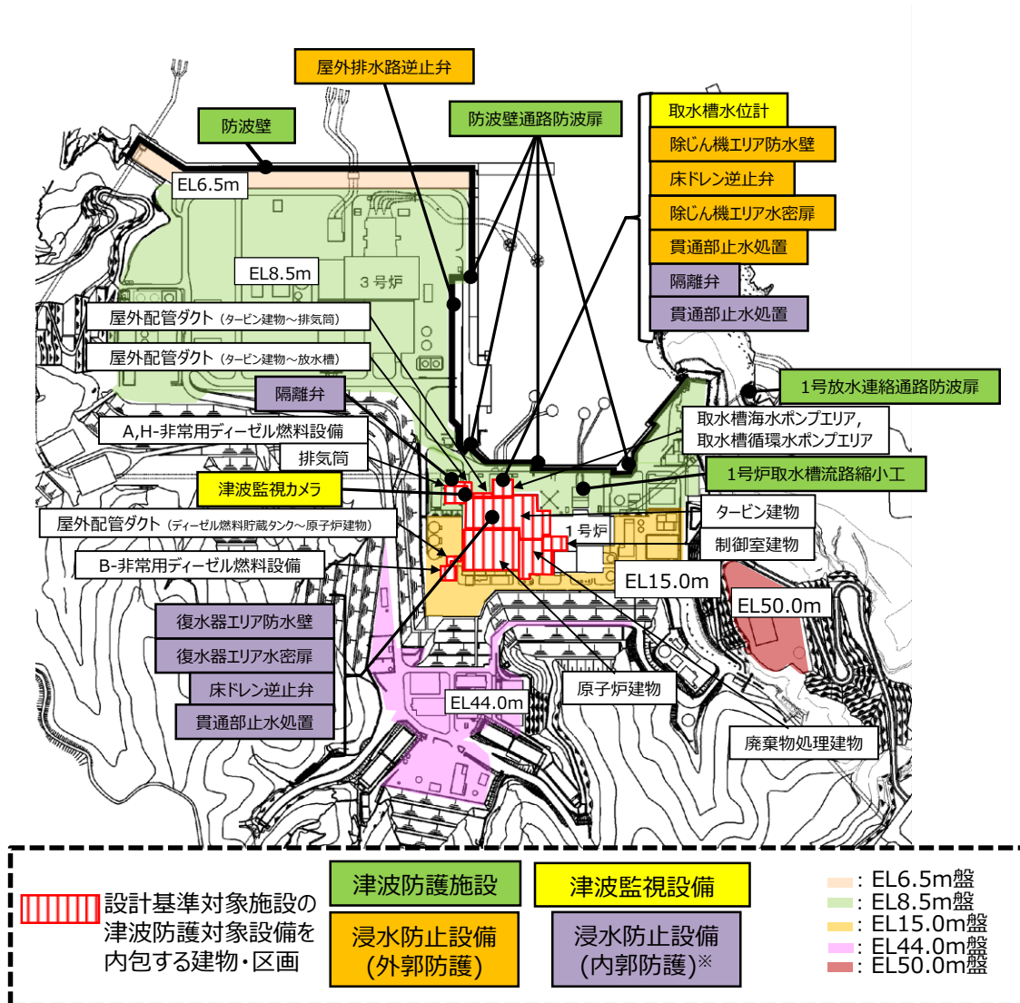
第 2.1-1 図 敷地の特性に応じた津波防護の概要
