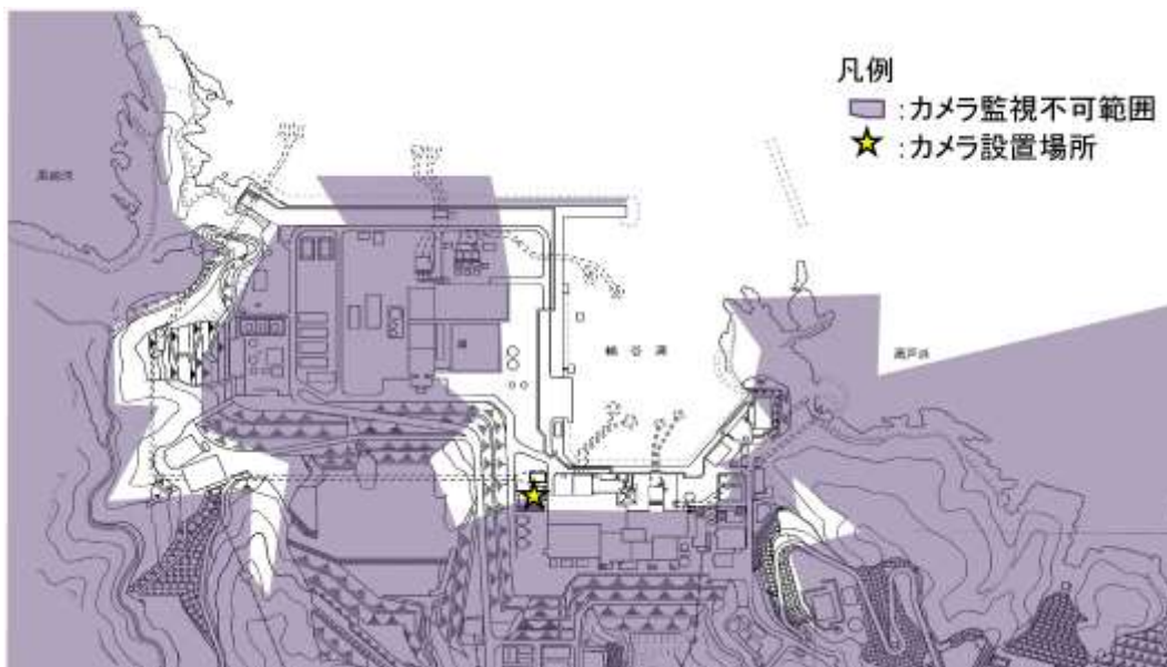
第4.3-4図 津波監視カメラの視野範囲
