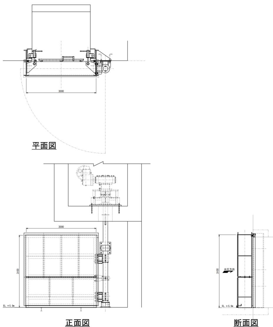
第 4.1-9 図 1号放水連絡通路防波扉構造図
