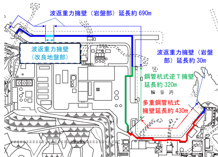
第 4.1-1 図 防波壁配置図
