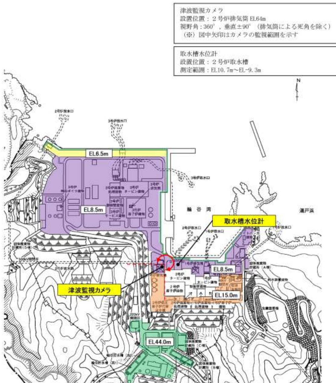
第4.3-1図 津波監視設備の配置
