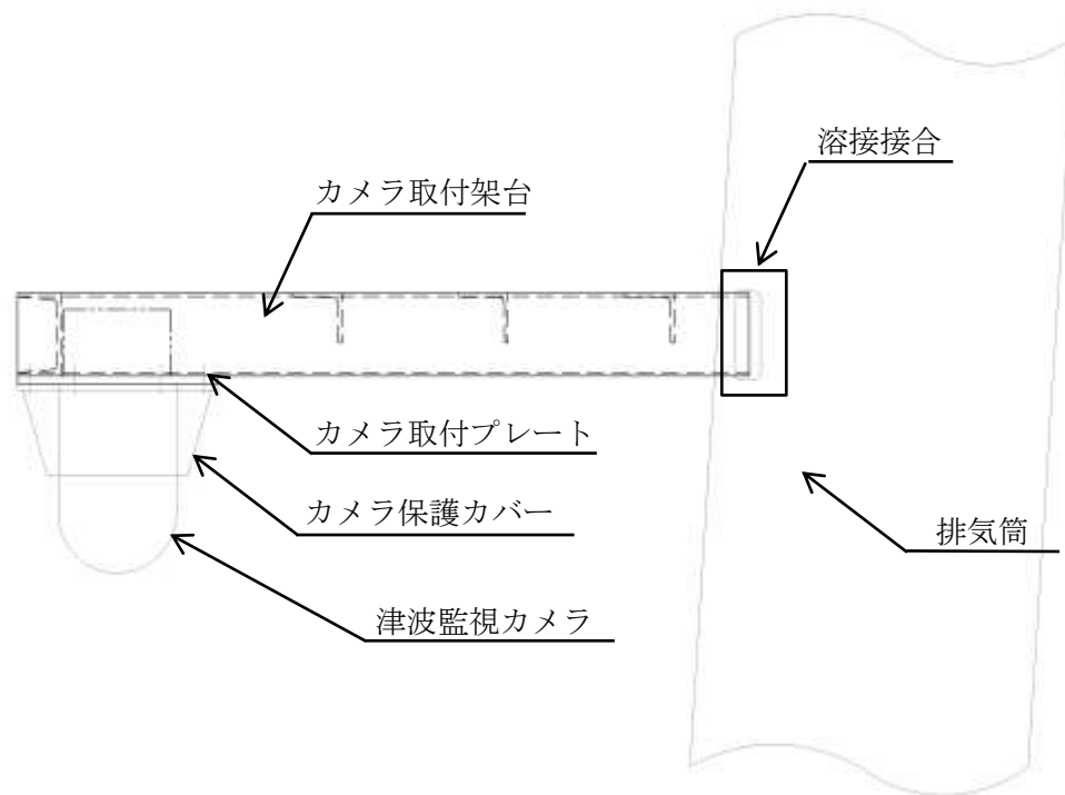
(断面図)
