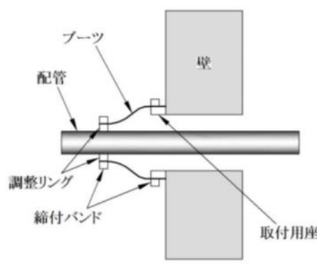
第10.6-16図 貫通部止水処置の概念図
