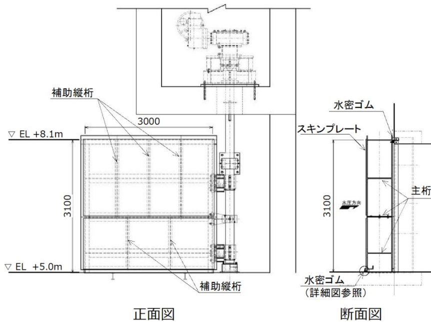
第10.6-6図 1号放水連絡通路防波扉概念図
