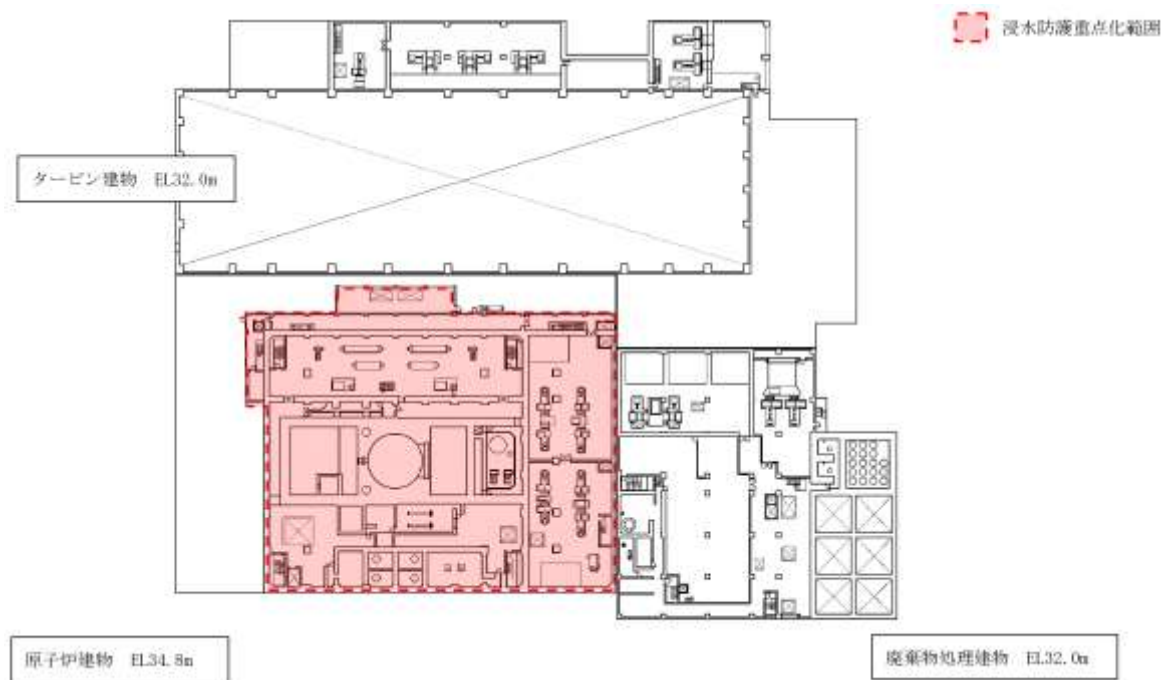
第 2.4-2-1 図 浸水防護重点化範囲（平面図）（3 / 4）
