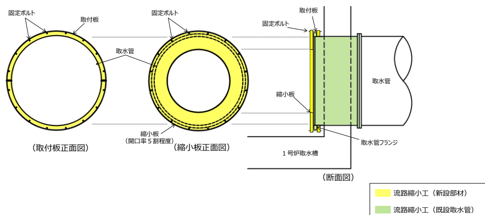
第4.1-11図 1号炉取水槽流路縮小工の構造例
