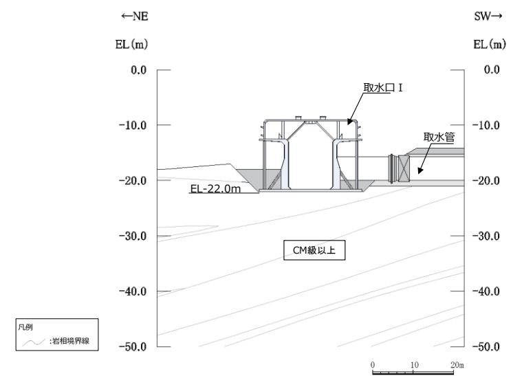
第6-2-11-7図 取水口 岩級断面図 (②-②断面)
