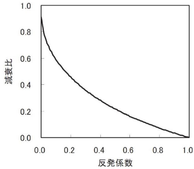
第1.3 図 反発係数と減衰比の関係
