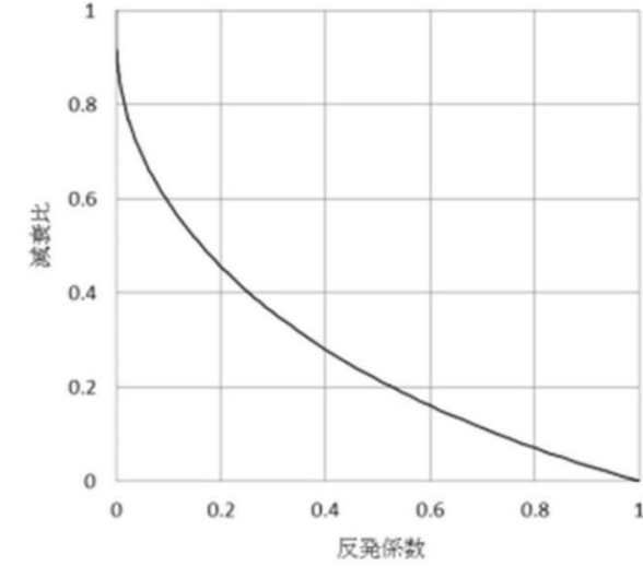
第 3-3 添図 反発係数と減衰比の関係
