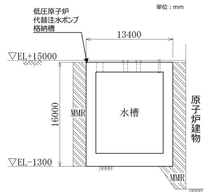
第6-2-4-5図 低圧原子炉代替注水ポンプ格納槽 断面図 (②)
