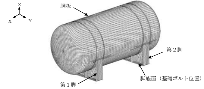
(1) 非常用ディーゼル発電設備ディーゼル燃料デイトンク
