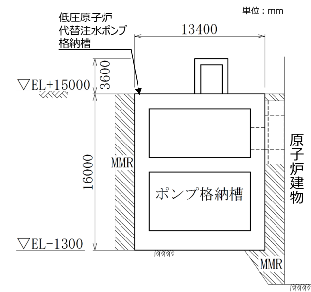
第6-2-4-4図 低圧原子炉代替注水ポンプ格納槽 断面図 (①)
