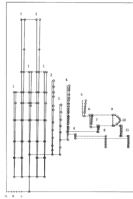
第2-2-1 図 (a) 影響検討モデル2 第1次振動モード図 (NS方向)
