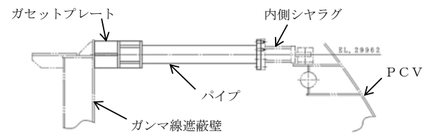
PCVスタビライザ構造図
