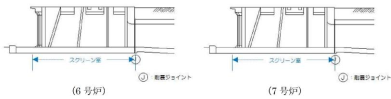
第12-1-4 図 6号及び7号炉スクリーン室 縦断面図
