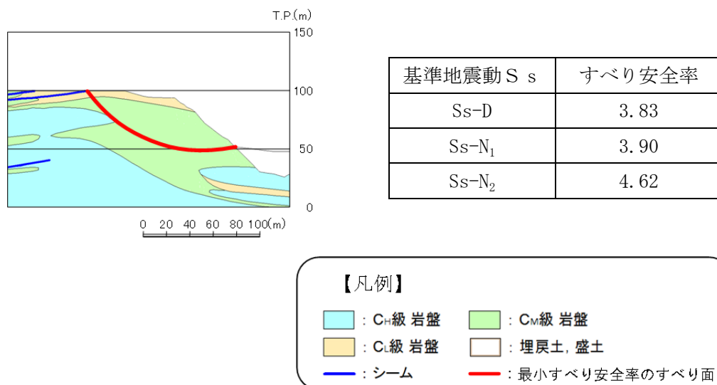
第 5.3-2 図 ⑩-⑩' 断面の評価結果
