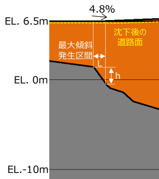
②-②断面
