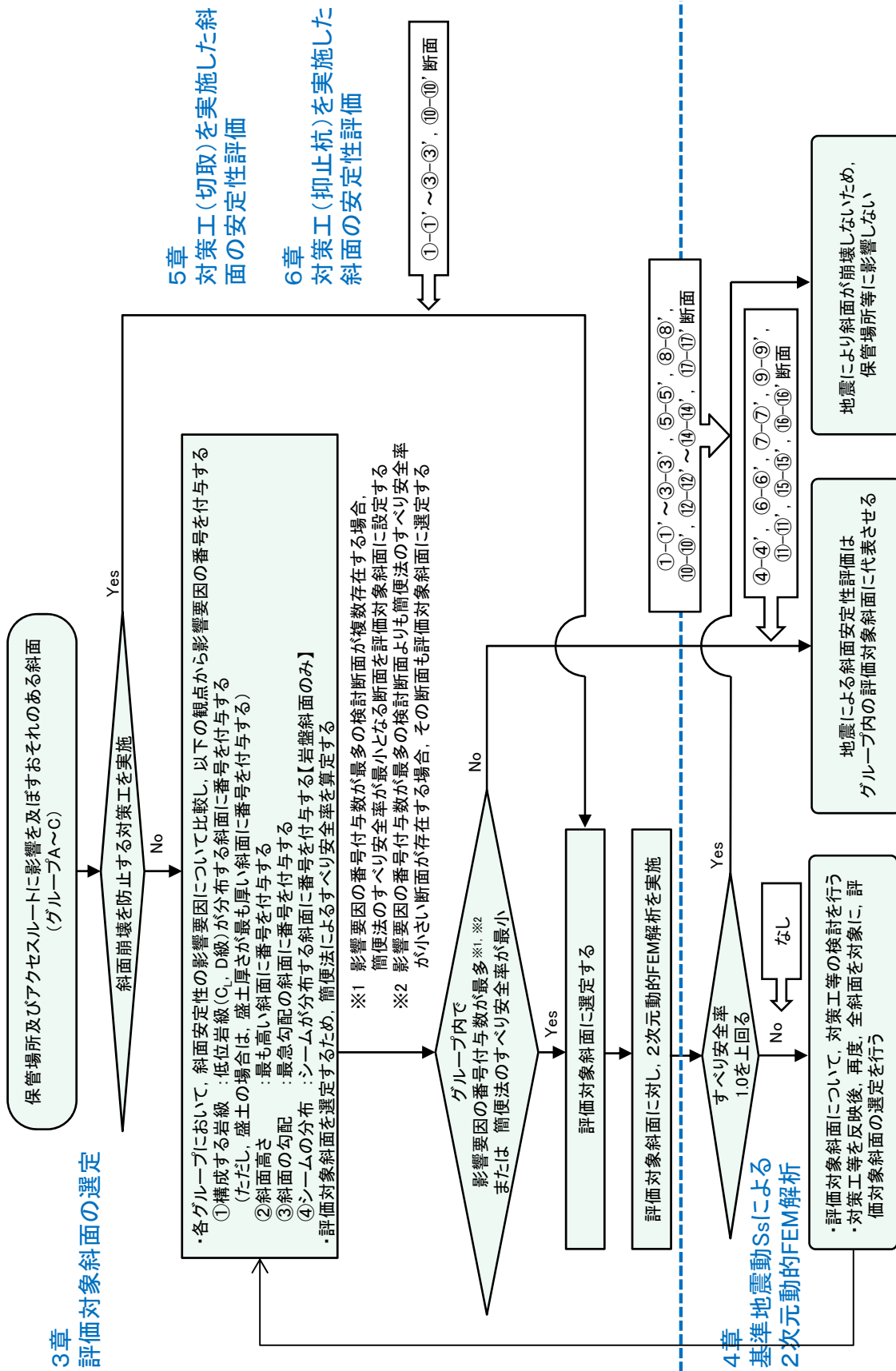
第3.1-1図 保管場所等の評価対象斜面のすべりに対する安定性評価のフロー
