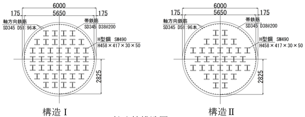
抑止杭構造図
