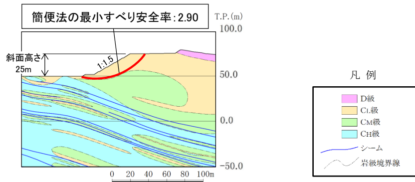
第 11 図 ⑩-⑩' 断面の比較結果
