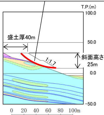
第6図 ⑨-⑨' 断面の比較結果
