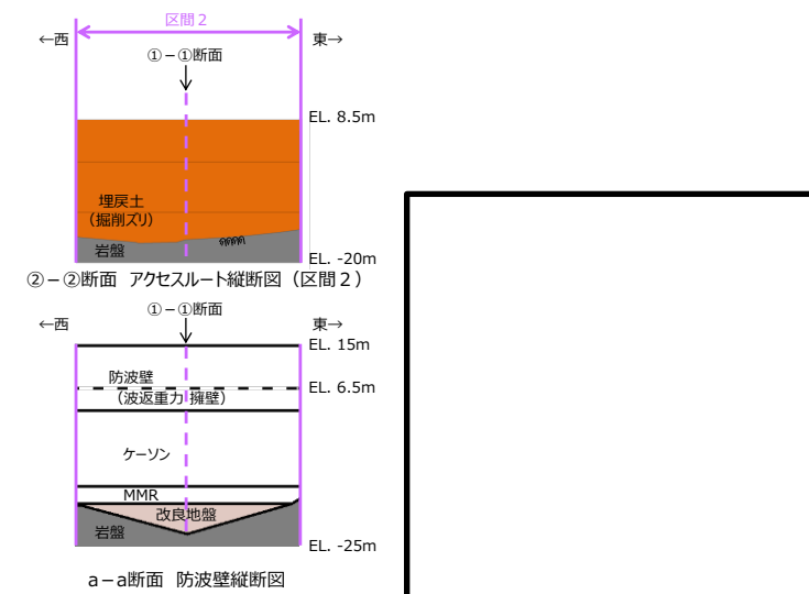
第 4-24 図 防波壁（波返重力擁壁）（縦断図）
