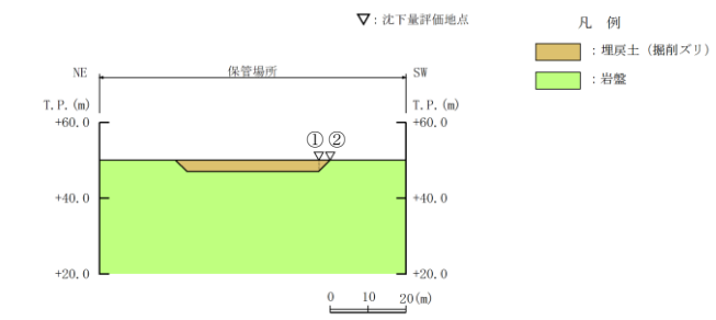
断面図
