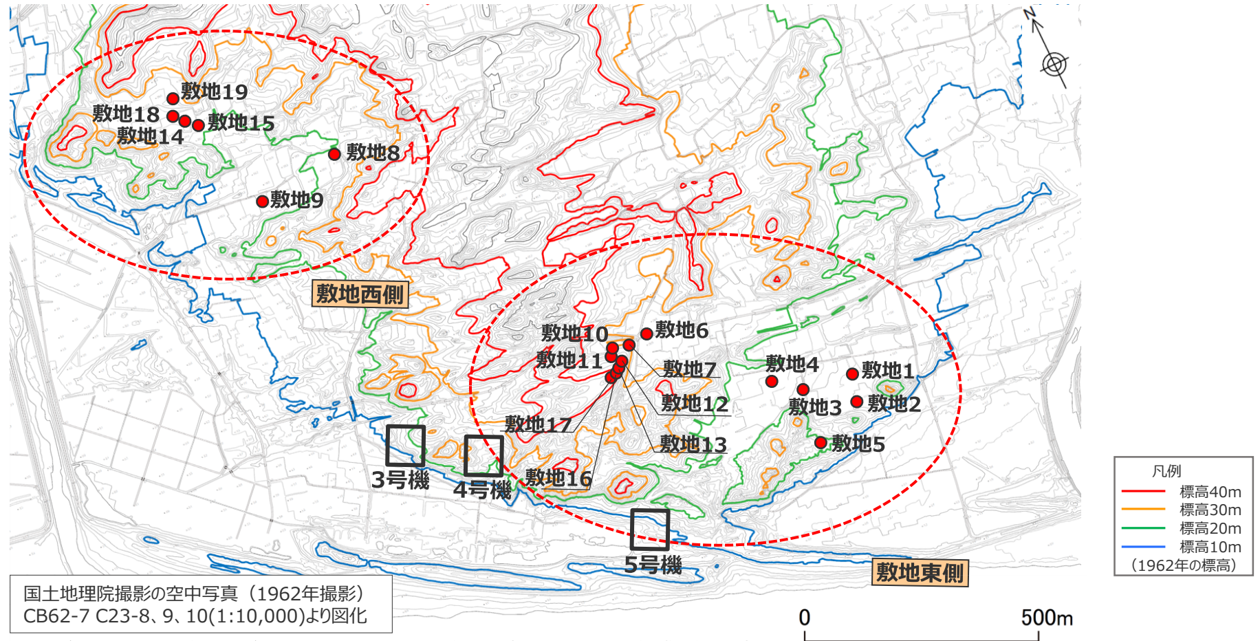
敷地のボーリング調査地点（発電所開発前の地形図に投影）
